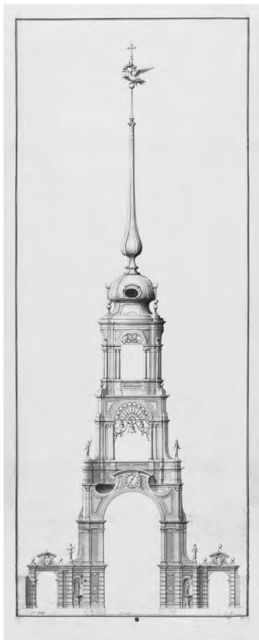
Ил. 4. Никола Микетти. Маяк в Кронштадте. Фасад. Проект. Италия. 1721–1722 г. Перо, кисть, тушь. Государственный Эрмитаж
