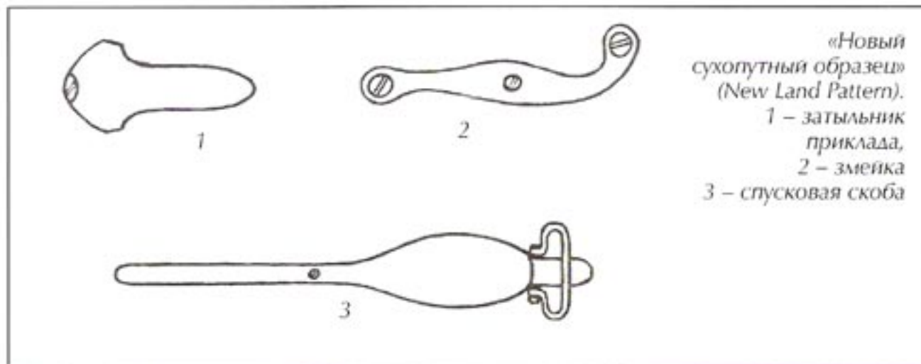
Модификации «Браун Бесс» легко отличить друг от друга по форме прибора. На фото слева приведён вид различных вариантов мушкета (слева направо) собственно «Браун Бесс», мушкет образца Ост-Индской компании и «Новый сухопутный образец». Справа приведена форма прибора различных вариантов мушкета
