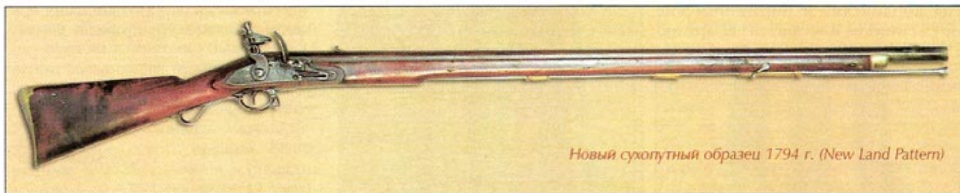
Мушкет образца Ост-Индской компании (India Pattern Musket)
