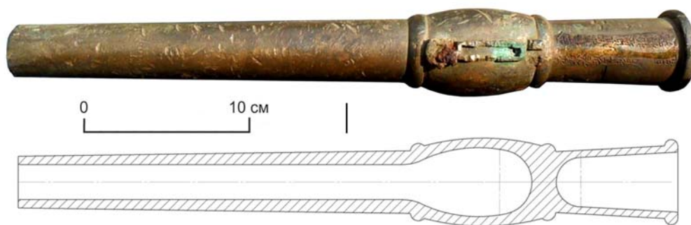
Рис. 1. Бронзовая китайская ручница из долины р. Джиды в Бурятии (фото Ю. В. Оборина)
