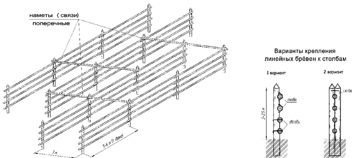
Рис. 1. Надолбы. Реконструкция автора.
