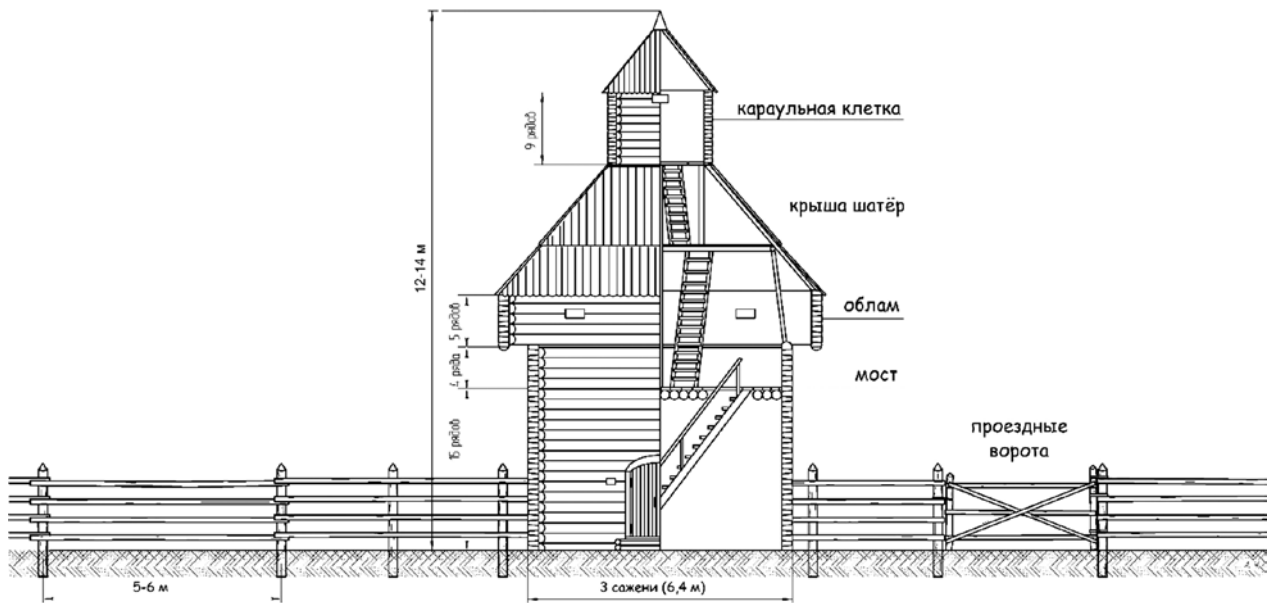
Рис. 2. Полевая сторожевая башня. Реконструкция автора.
