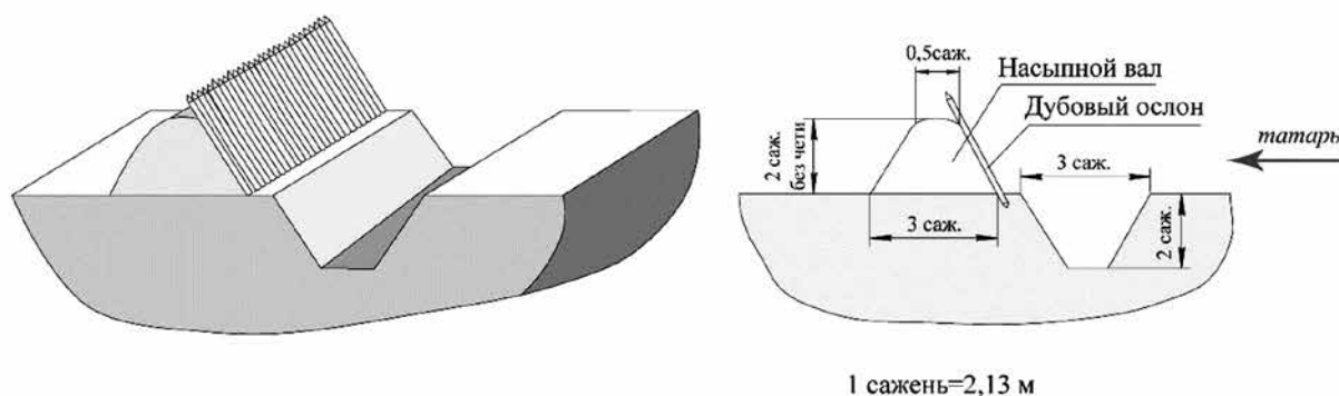
Рис. 1. Чертёж защитного земляного вала XVII в.
