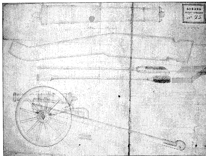
Чертеж 24-фунтовой пушки, выполненный Я.У. Шперрейтером. Вторая четверть XVIII в.
