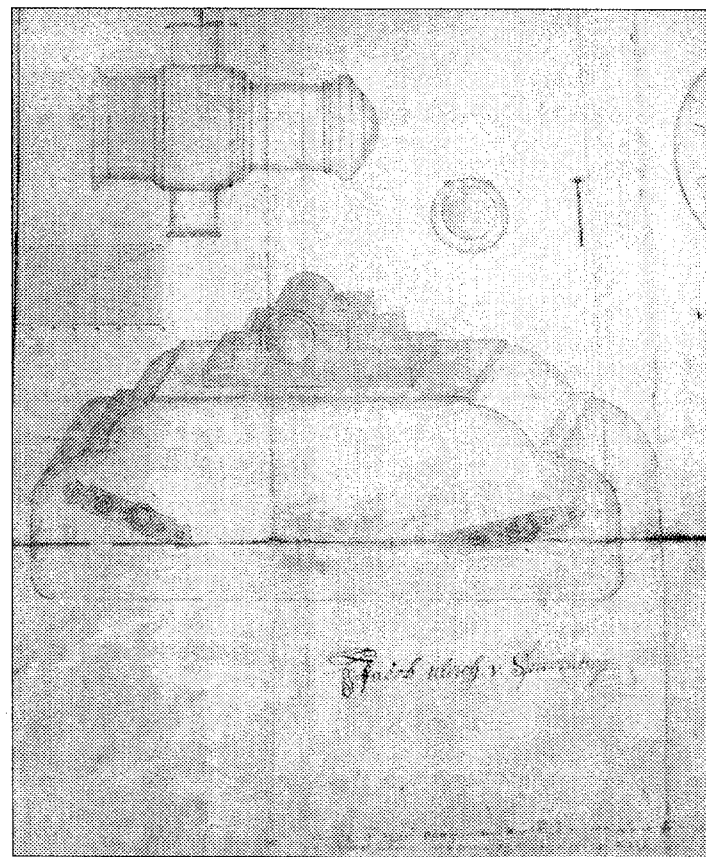
Чертеж мортиры, выполненный Я.У. Шперрейтером. Вторая четверть XVIII в.
