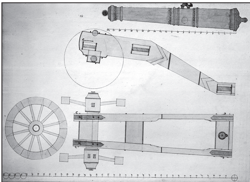
Чертеж 6-фунтовой полевой пушки на лафете. Первое десятилетие XVIII в. Архив ВИМАИВиВС. Ф. 27. Оп. 15. Д. 41. Л. 31
