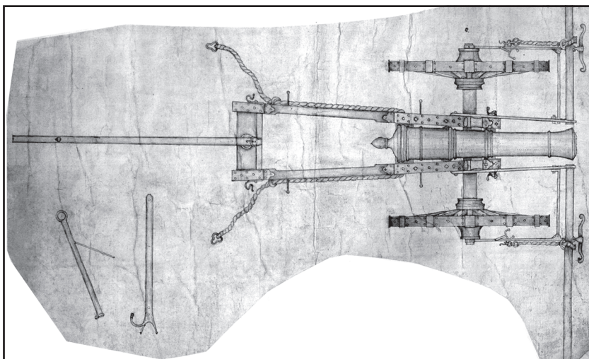
Чертеж 3-фунтовой полевой пушки на лафете. Первое десятилетие XVIII в. Архив ВИМАИВиВС. Ф. 27. Оп. 15. Д. 41. Л. 34
