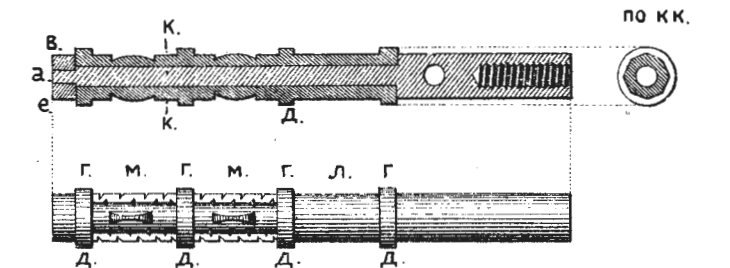
Рис.258. Протирка.
