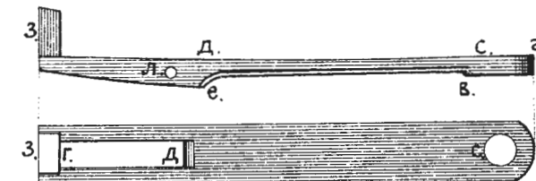
Рис. 92. Пружина.
