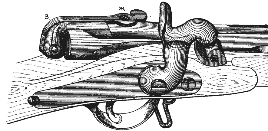
Рис.84. Затворъ закрытъ.
