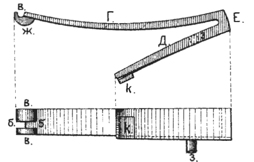
Рис.158.Боевая пружина.
