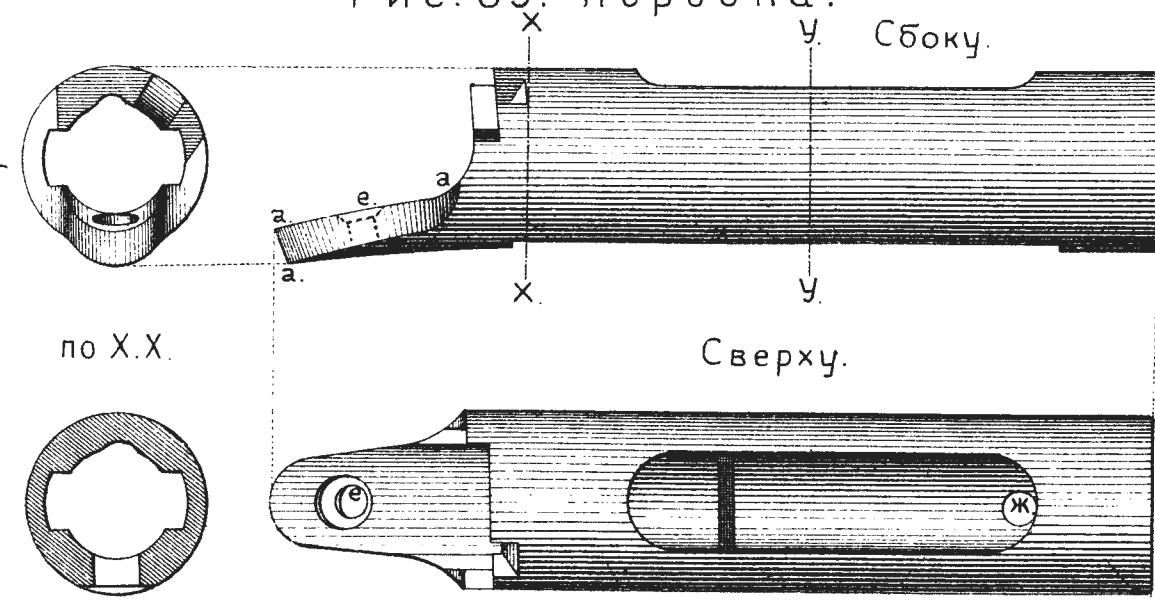
Рис. 89. Коробка.
