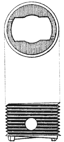
Рис.85. Кольцо затвора.
