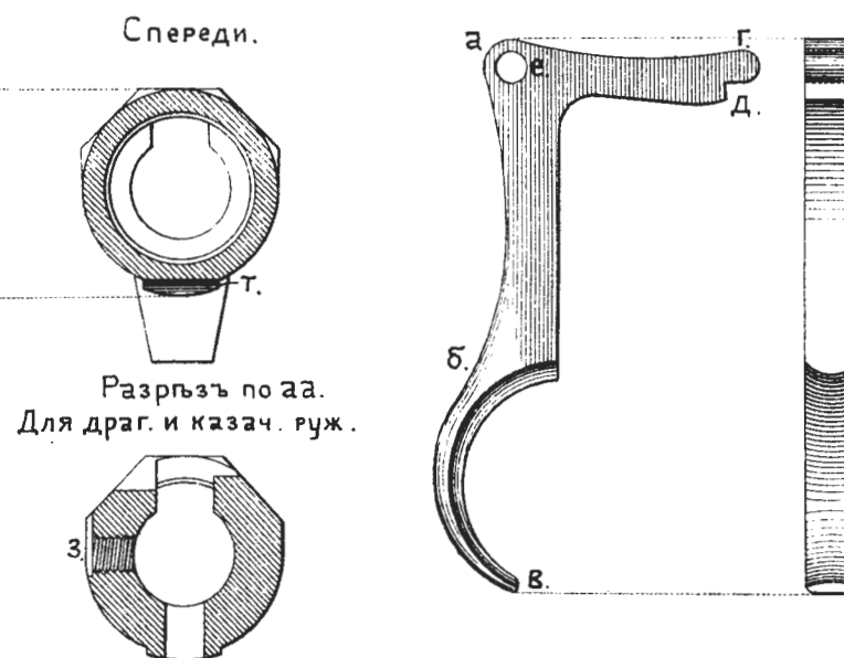
Рис.206. Спускъ пѣхотный.
