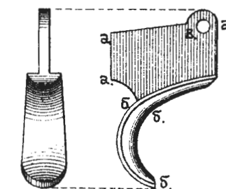
Рис. 110. Спускъ.
