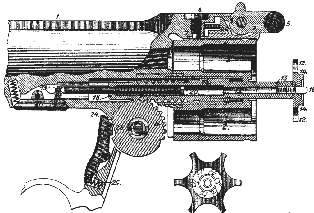
Рис.271. Револьверъ открытъ.
