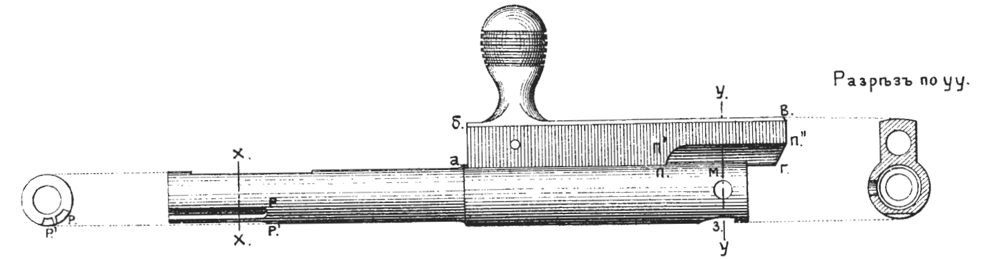
Рис.221. Стебель затвора.
