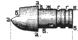
Рис.150.Боекъ. Рис.149.Винтъ бойка.
