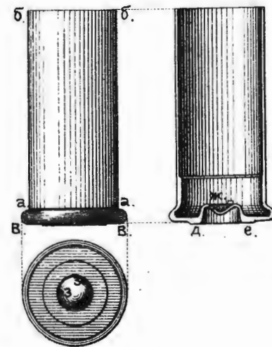
Рис.165. Гильза
