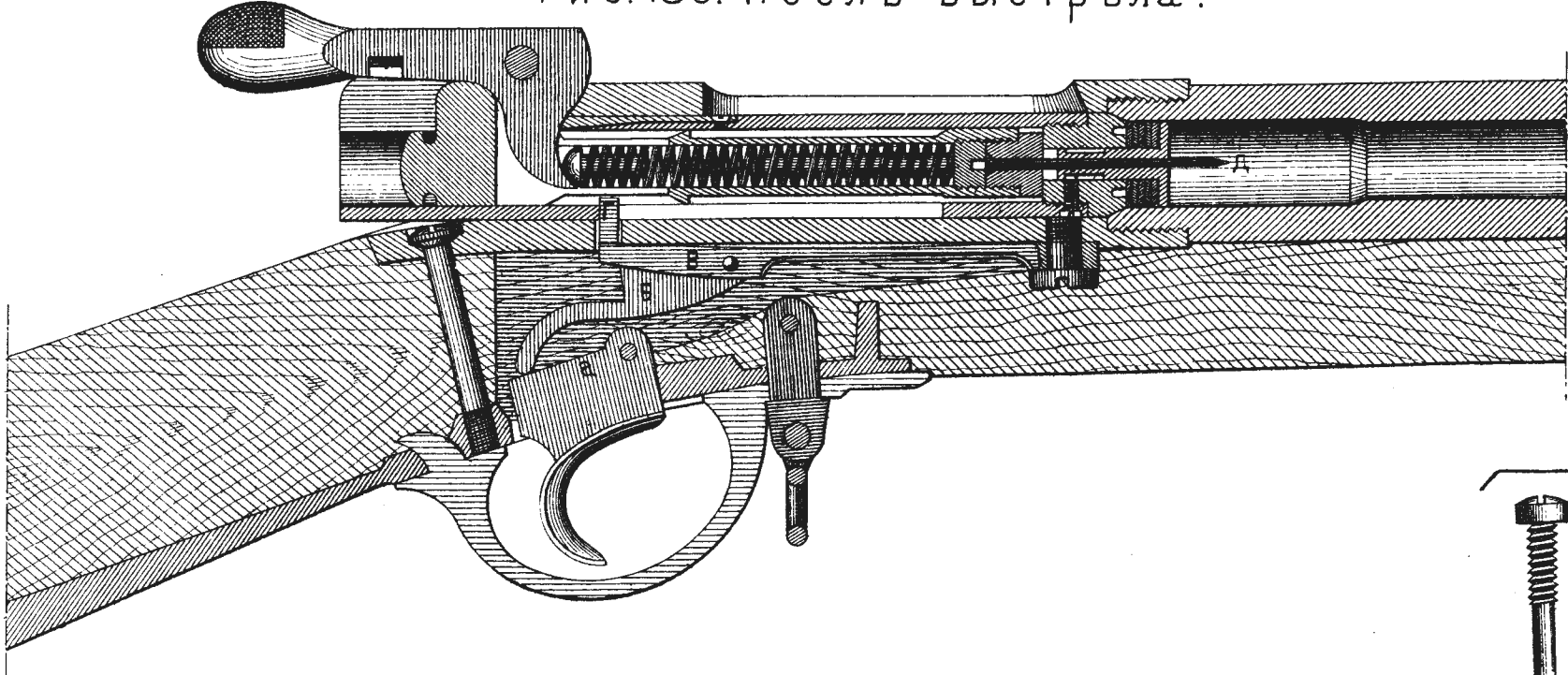
Рис. 130. Послѣ выстрѣла.
