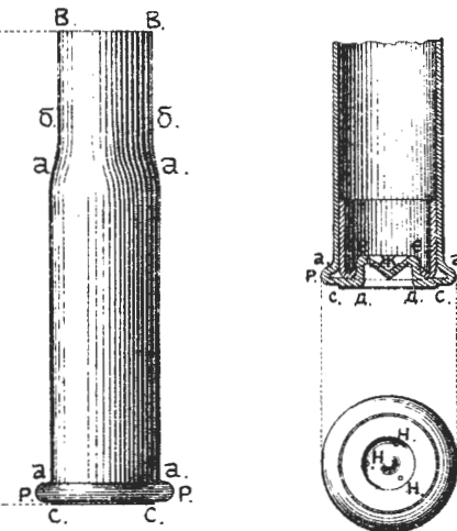
Рис.266. Просальникъ
