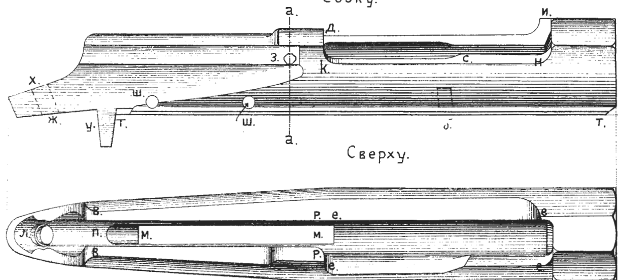
Рис.205. Коробка Сбоку.
