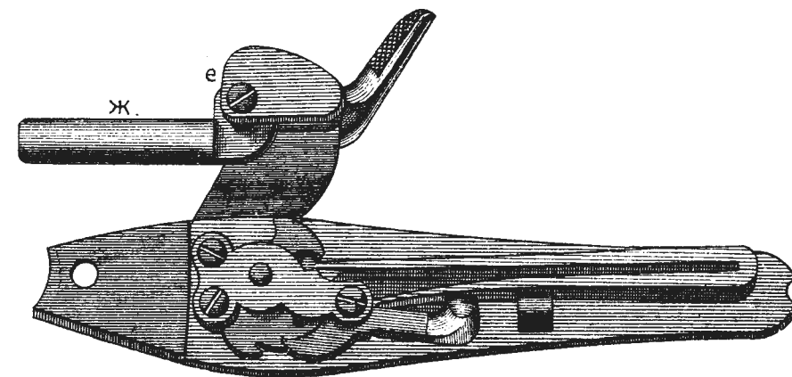
Рис.137. Замокъ.
