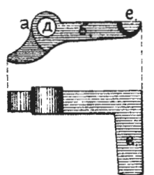
Рис.160.Крючекъ.
