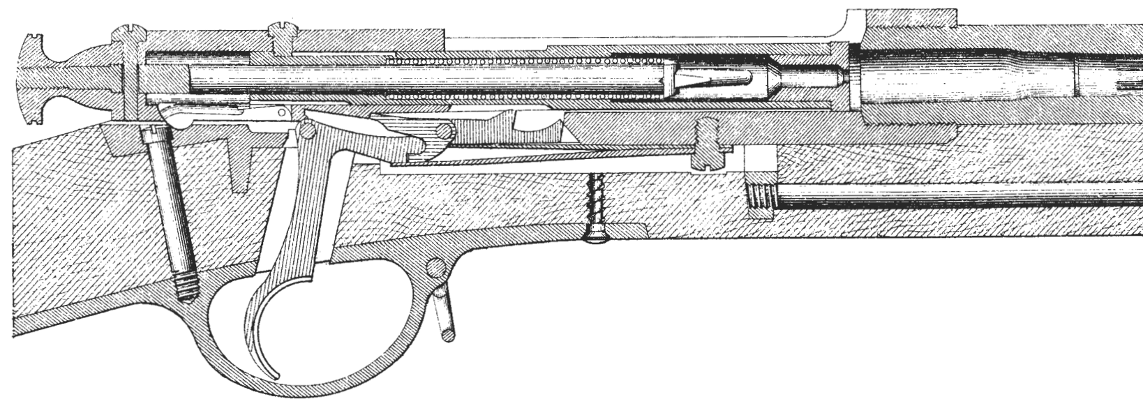
Рис.261. Напредохранител. взводѣ.
