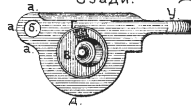
Рис.148.Затворъ съ бойкомъ и ударникомъ.
