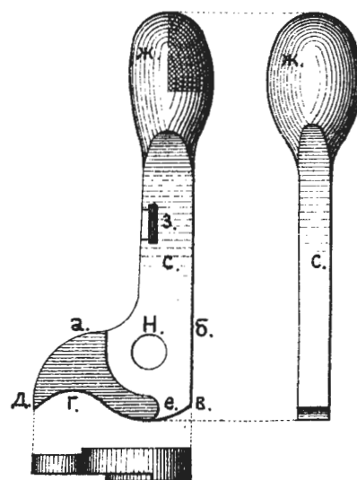
Рис. 99. Рукоятка.
