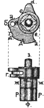
Рис.155.Ладыжка.
