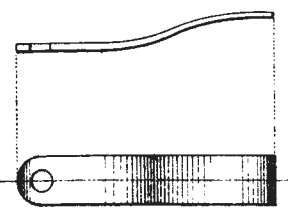
Рис.176. Подстрѣлочная пружина.
