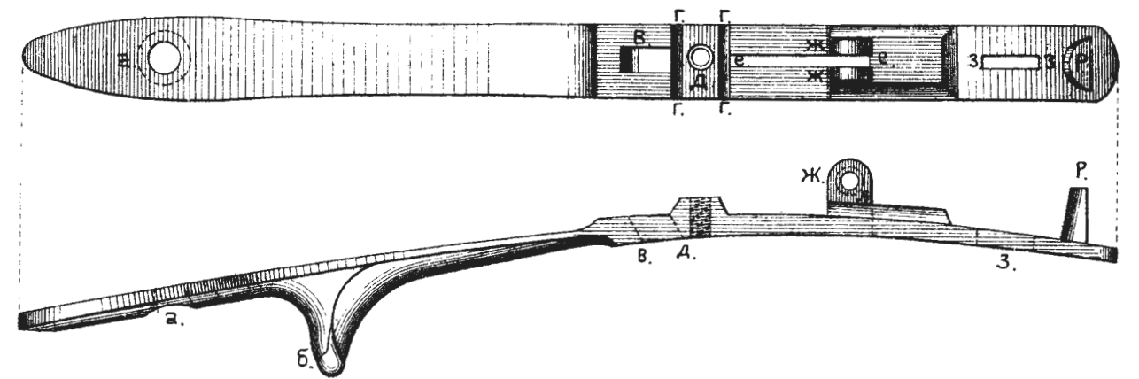
Рис.123. Спускъ личинка.
