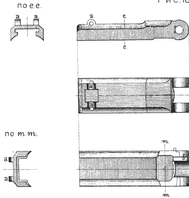
Рис.180. Стрѣлка.
