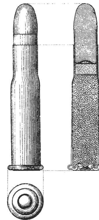
Рис.262. Боевой патр. къ винтовкѣ Бердана №2
