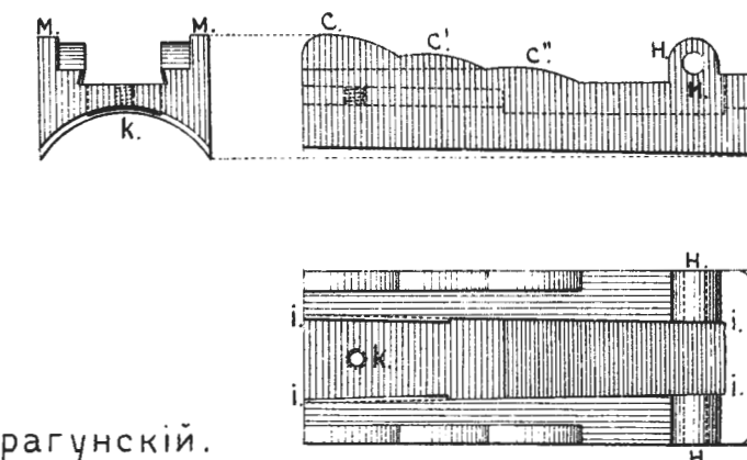
Рис.201. Прицѣльная колодка
