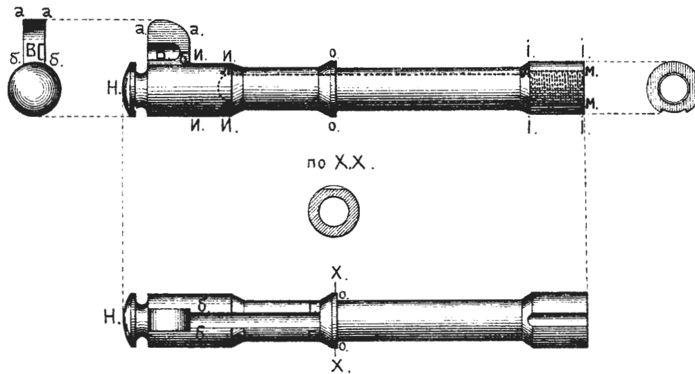
Рис. 104. Стебель ударника.
