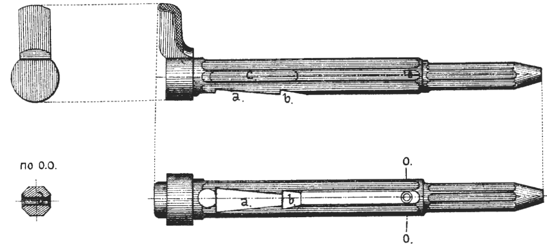
Рис.187. Курокъ.
