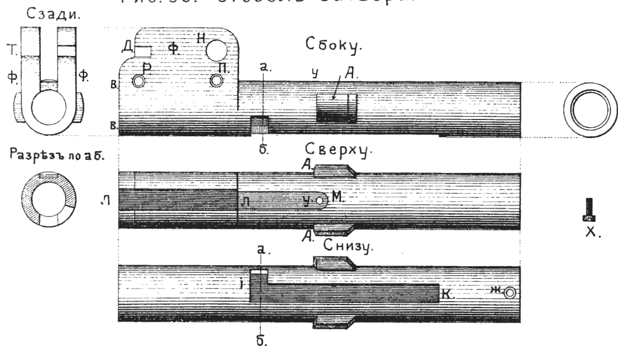
Рис. 96. Стебель затвора.
