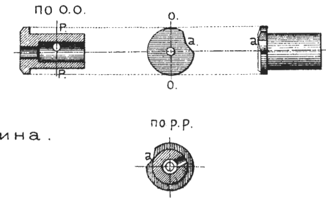
Рис.182. Личинка.
