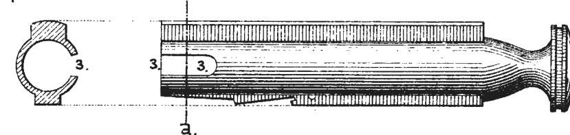
Рис.232. Положеніе прорѣза для драгунск. и казач.винт.
