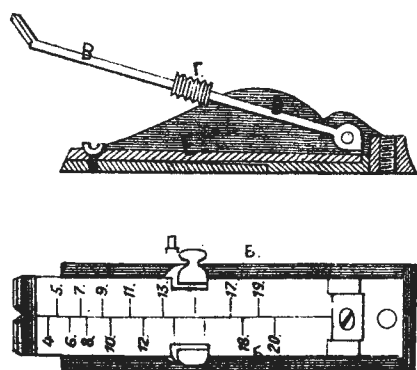
Рис.274. Прицѣль къ кръпостному ружью.
