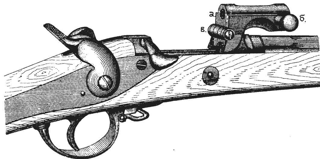
Рис.135. Затворъ открытъ.
