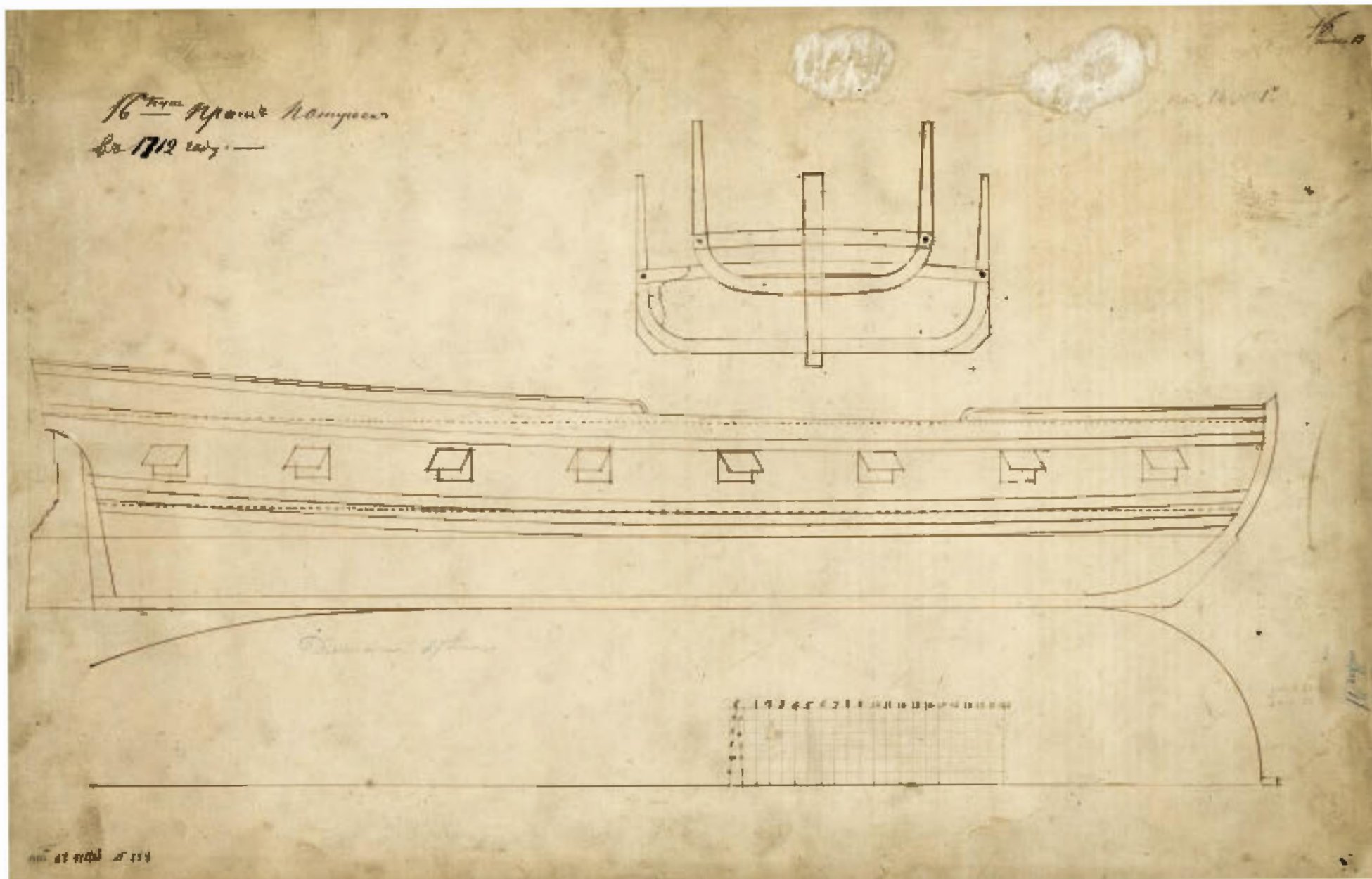
Чертеж 16-ти пушечного прам (плоскодонное судно, вооруженное пушками крупного калибра). 1712 г.
