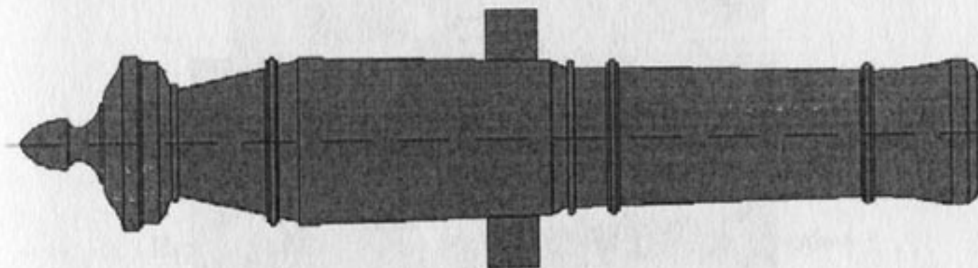
Рис. 1. Российский 3-фунтовый единорог системы 1805 года с изменениями 1812 года, вид сверху. Схема создана на основании чертежей, опубликованных А. И. Маркевичем и В. К. Плотто
