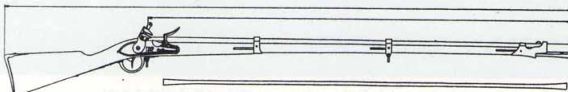
Karabin piechoty wzór 1826
