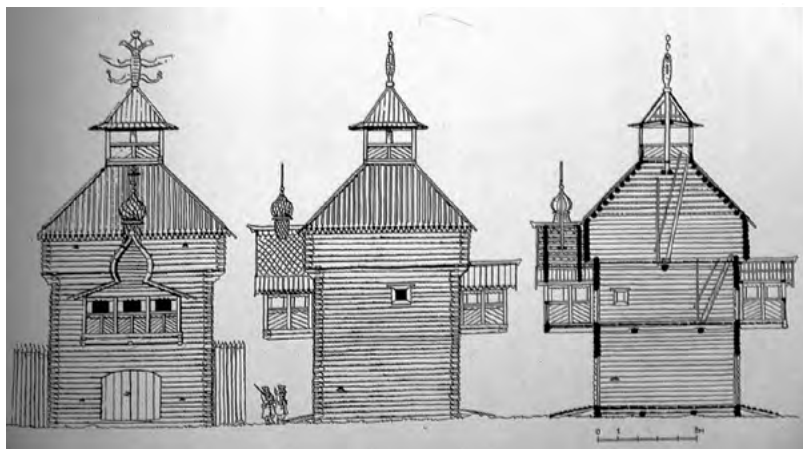
Рис. 7. — Илимский острог 1694 г. Воротная башня. Реконструкция двух фасадов и разреза на основе фиксационных обмеров. Н.П. Крадин
