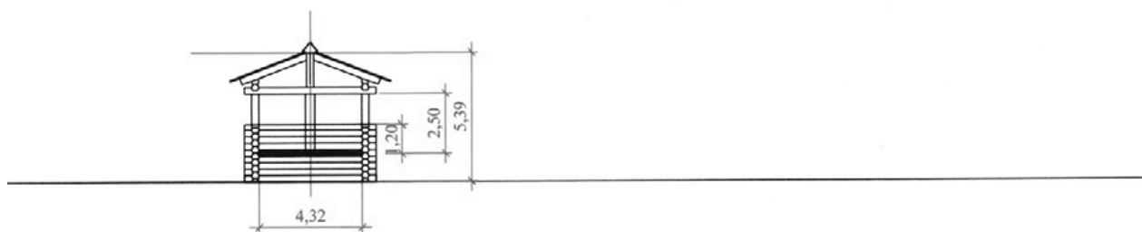
Рис. 8. — Холмогорская крепость. Разрезы двух прясел. Реконструкция по росписи 1692 г. М.И. Мильчик, Н.А. Демченко.
