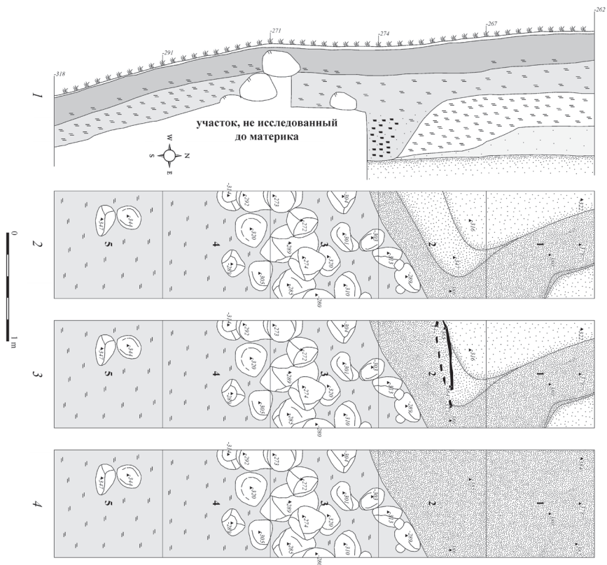
Рис. 16. Мядельский замок 2014. Планы и западный профиль Шурфа I (рис. автора)
