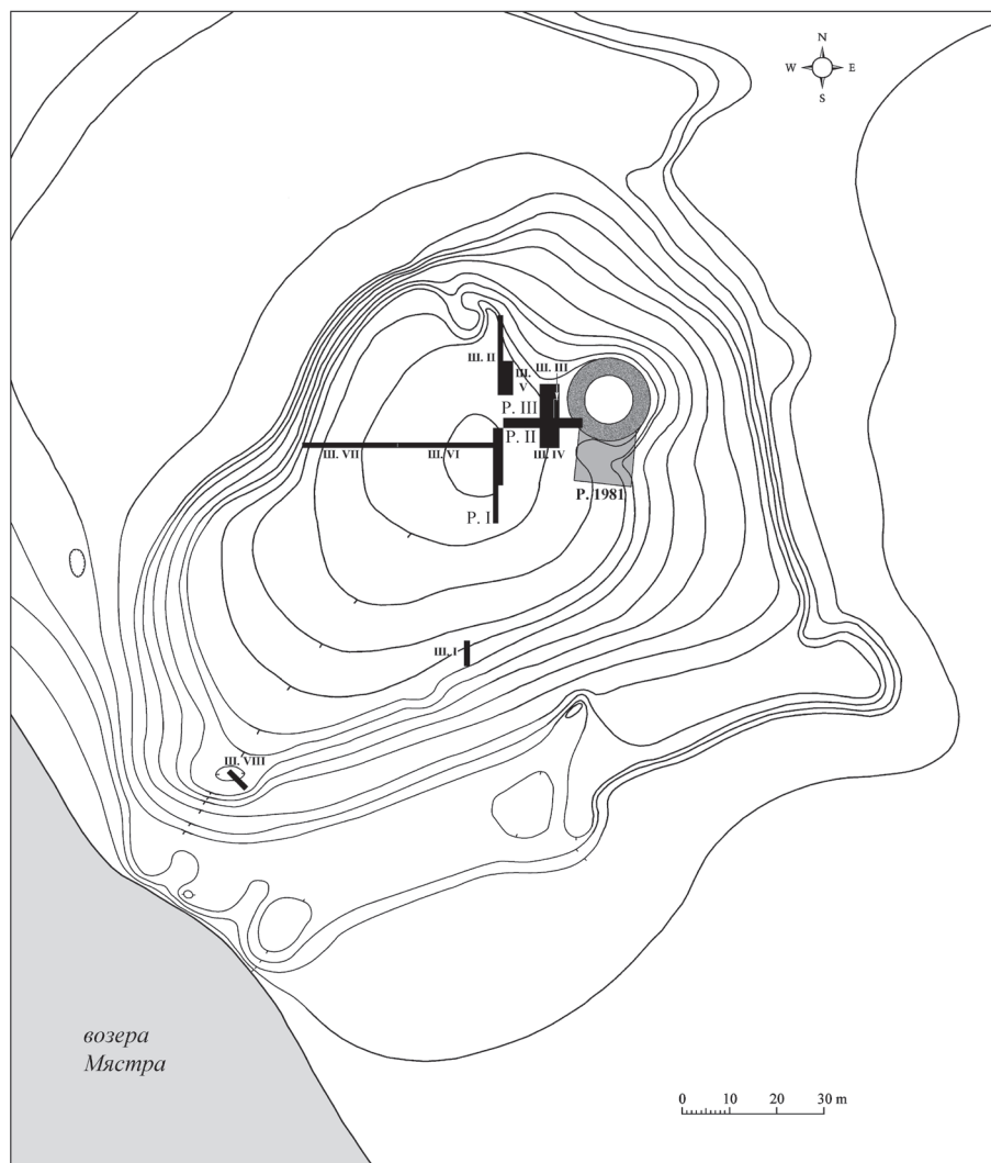
Рис. 5. План Мядельского замка (съёмка Э.А. Астаповича 2013 г.) с обозначением башни, раскопов и шурфов 2013–2015 гг. и приблизительного места расположения раскопа 1981 г.
