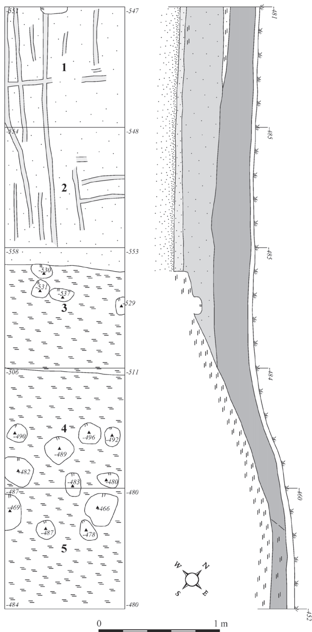
Рис. 19. Мядельский замок, 2015 г. План и профиль Шурфа VIII (рис. автора)
