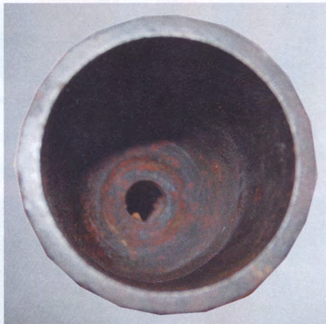
ВНУТРЕННЯЯ ЧАСТЬ СТВОЛА АНГЛИЙСКОЙ МОРТИРКИ. ХОРОШО ВИДНО ВЫХОДНОЕ ОТВЕРСТИЕ ОГНЕПРОВОДНОЙ ТРУБКИ
