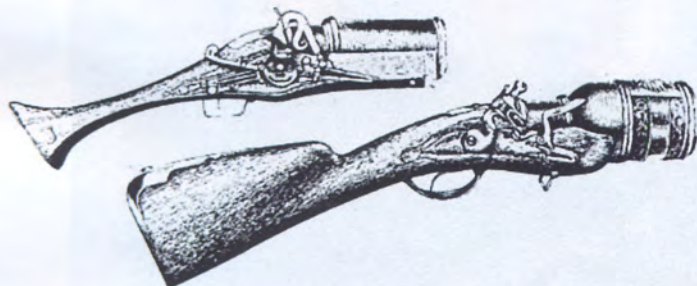
ТИПЫ РУЧНЫХ МОРТИРОК, КОТОРЫМИ БЫЛИ ВООРУЖЕНЫ АРМИИ ЗАПАДНО-ЕВРОПЕЙСКИХ СТРАН
