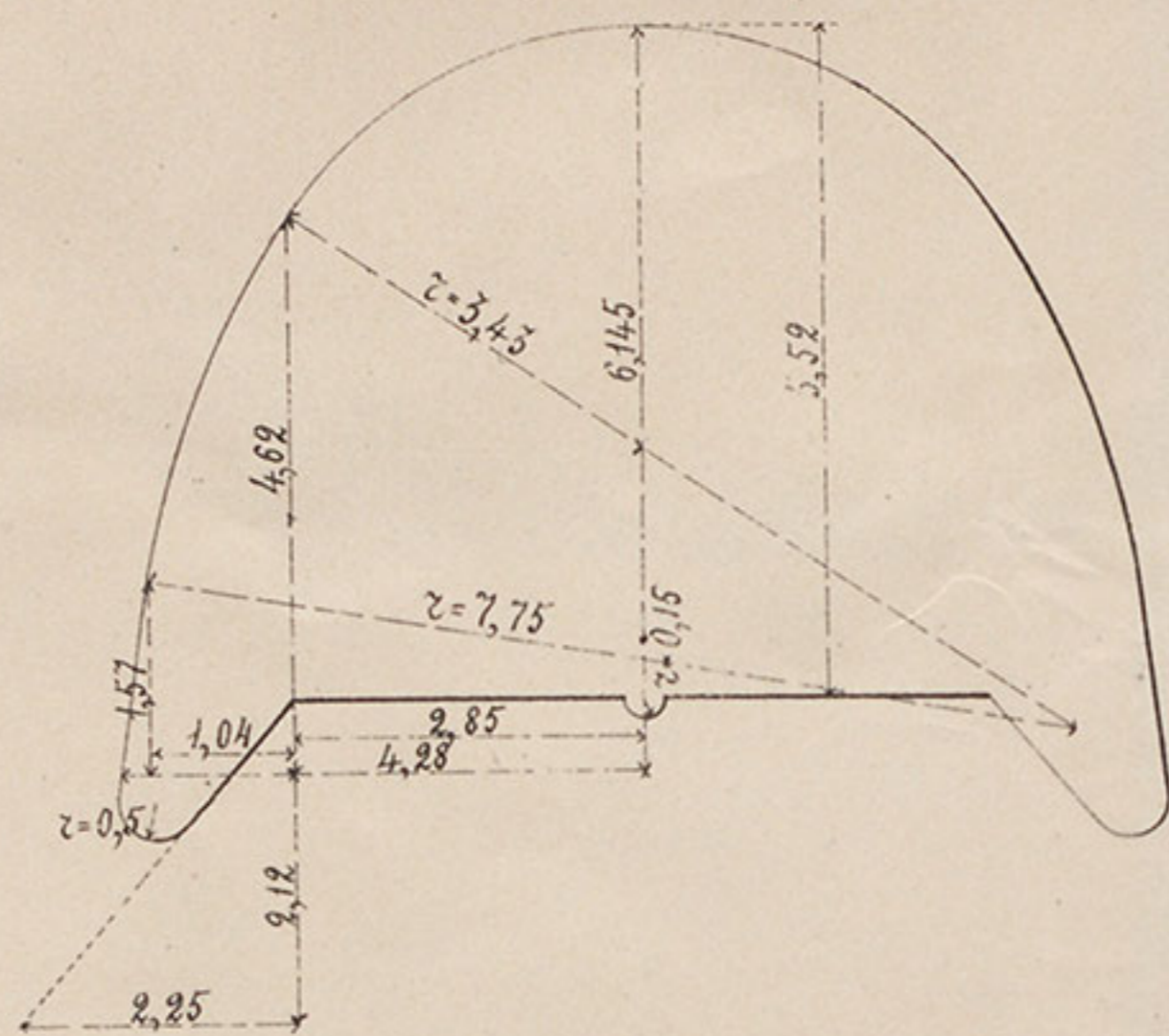
а. Пластина къ лекалу К.
