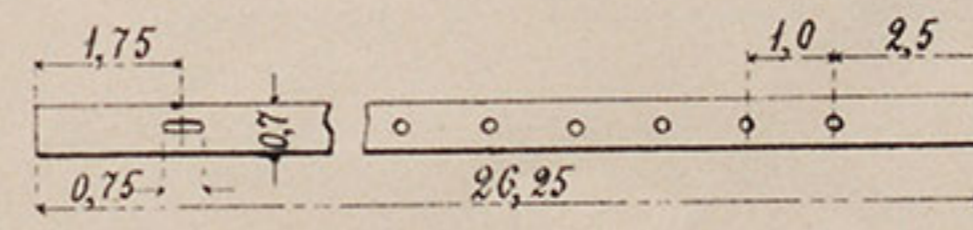
№ 90. Ремень для задняго средняго вьючнаго ремня.
