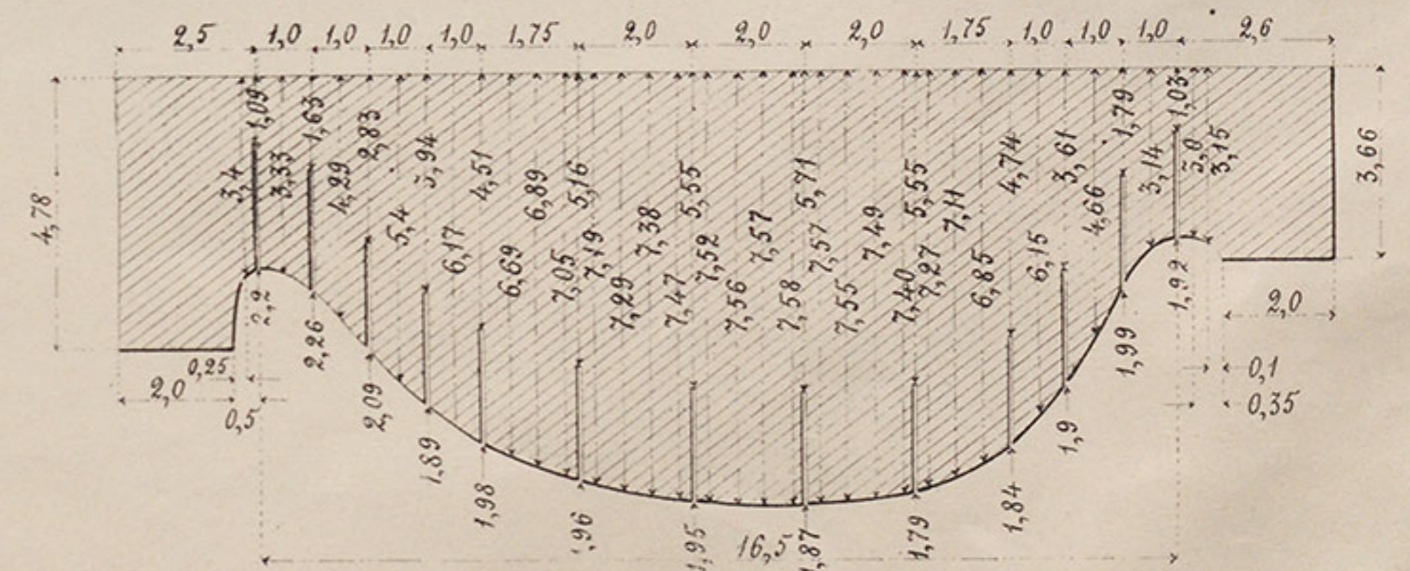
Лекало для сѣченія № II.
