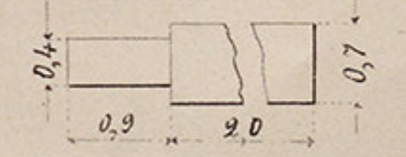
№ 52. Ремень для костылька.
