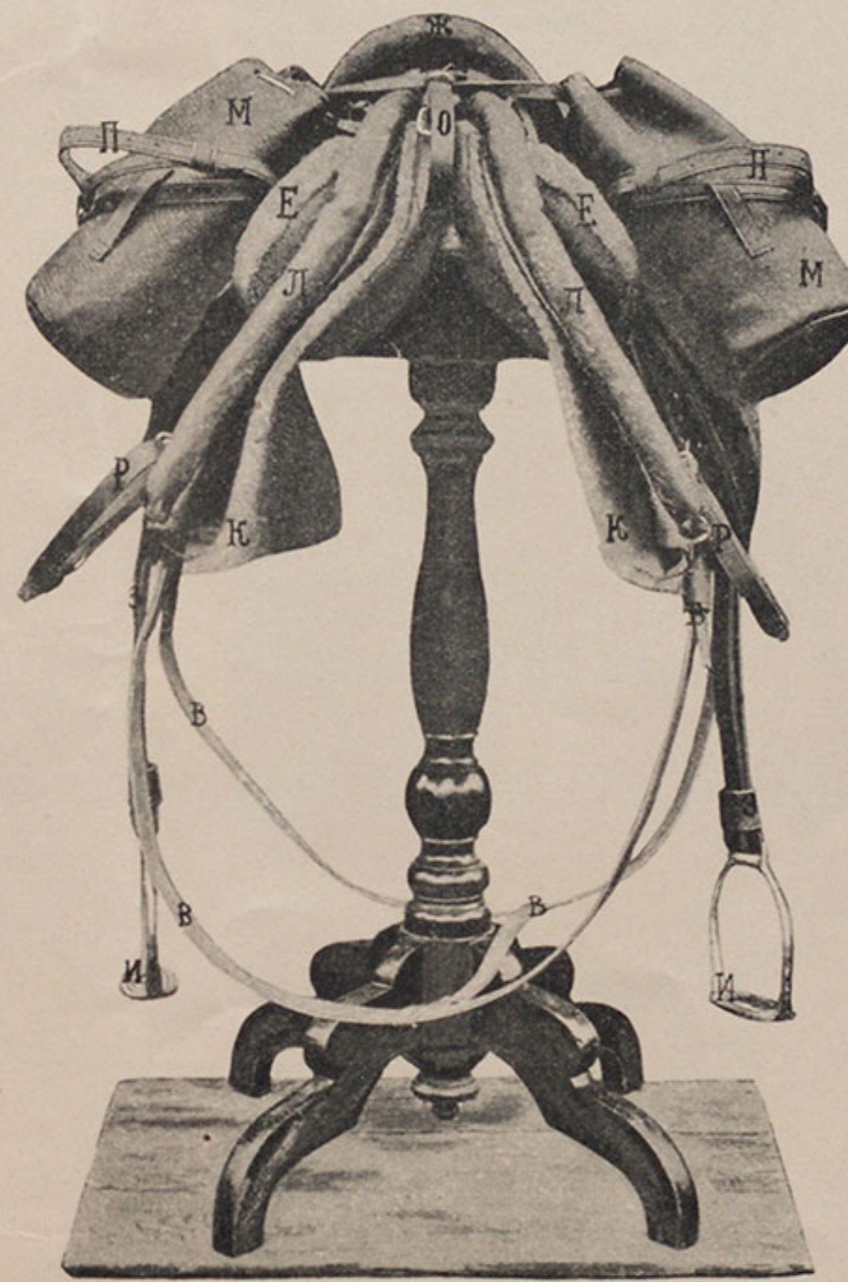
Видъ спереди.
