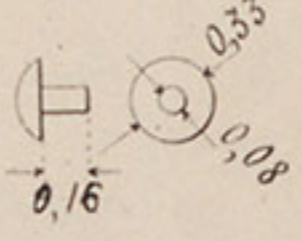
№ 44. Заклепка.
