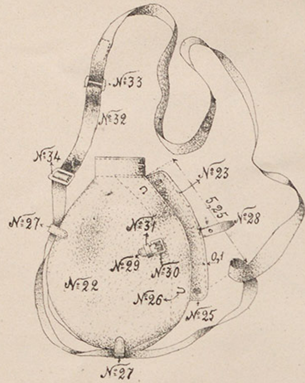
К. Чахолъ на флягу.
