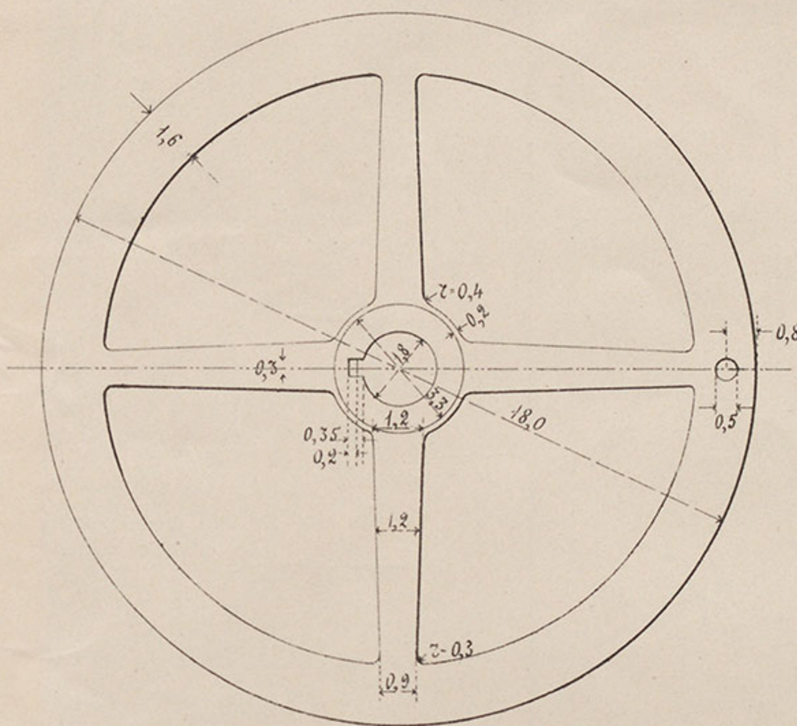
№ 14. Маховикъ.
