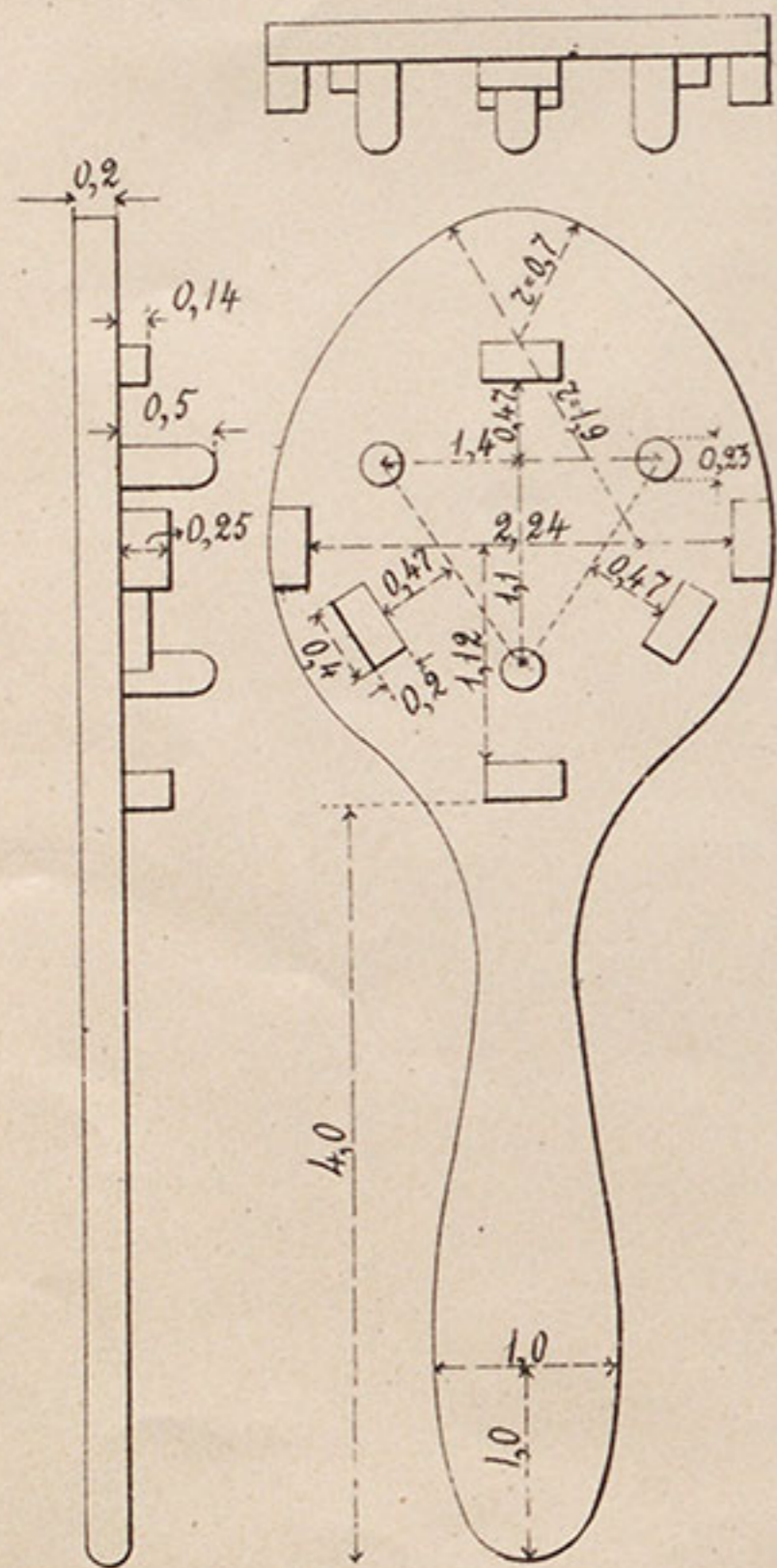
І. Лекало для повѣрки отверстій въ лапкахъ и планкахъ № 8.
