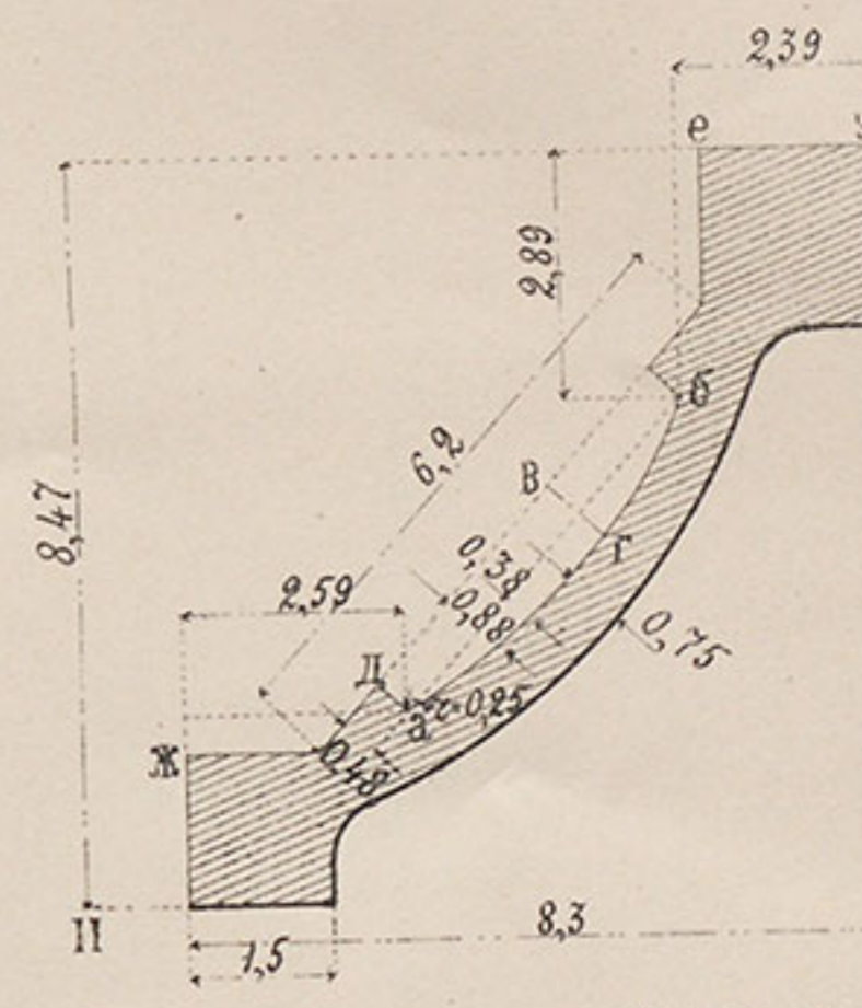
Г. Лекало для повѣрки отверстія для путлища.
