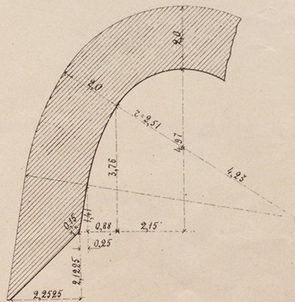
№ 46. Лекало къ станку Е.
