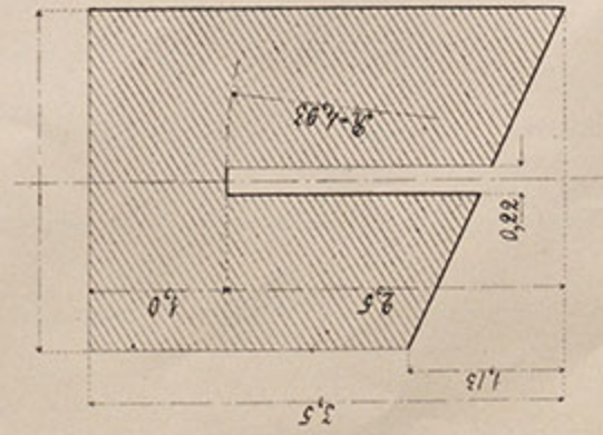
№ 58. Лекало къ станку.
