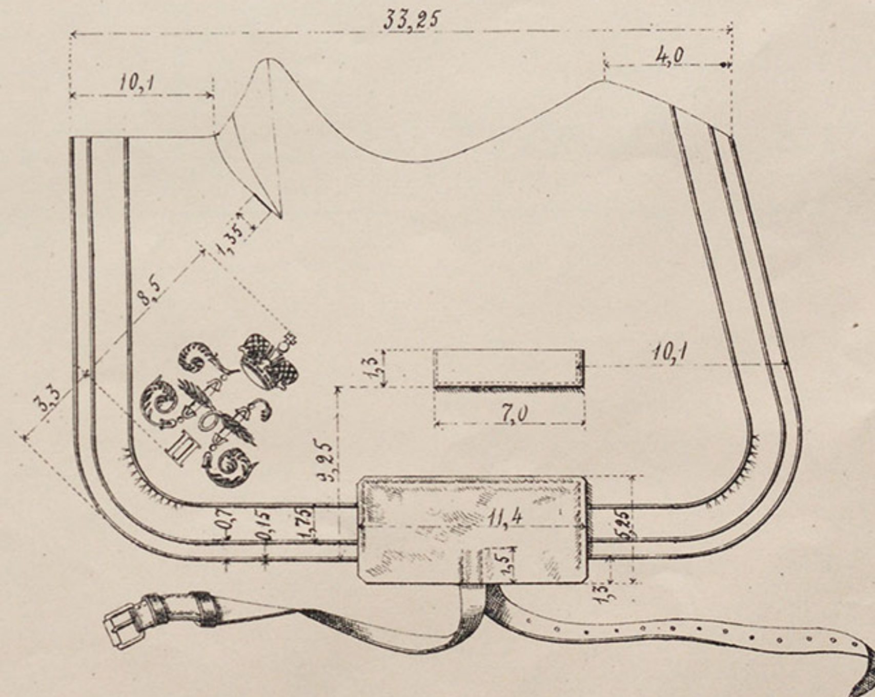
Обще-кавалерійскій вальтрапъ.
