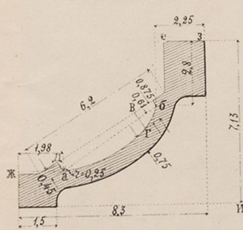
Пластика для сѣченія № 6.
