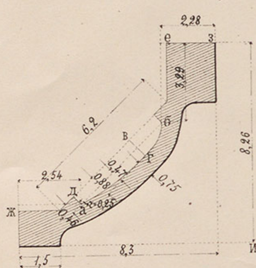
Пластика для сѣченія № 3.
