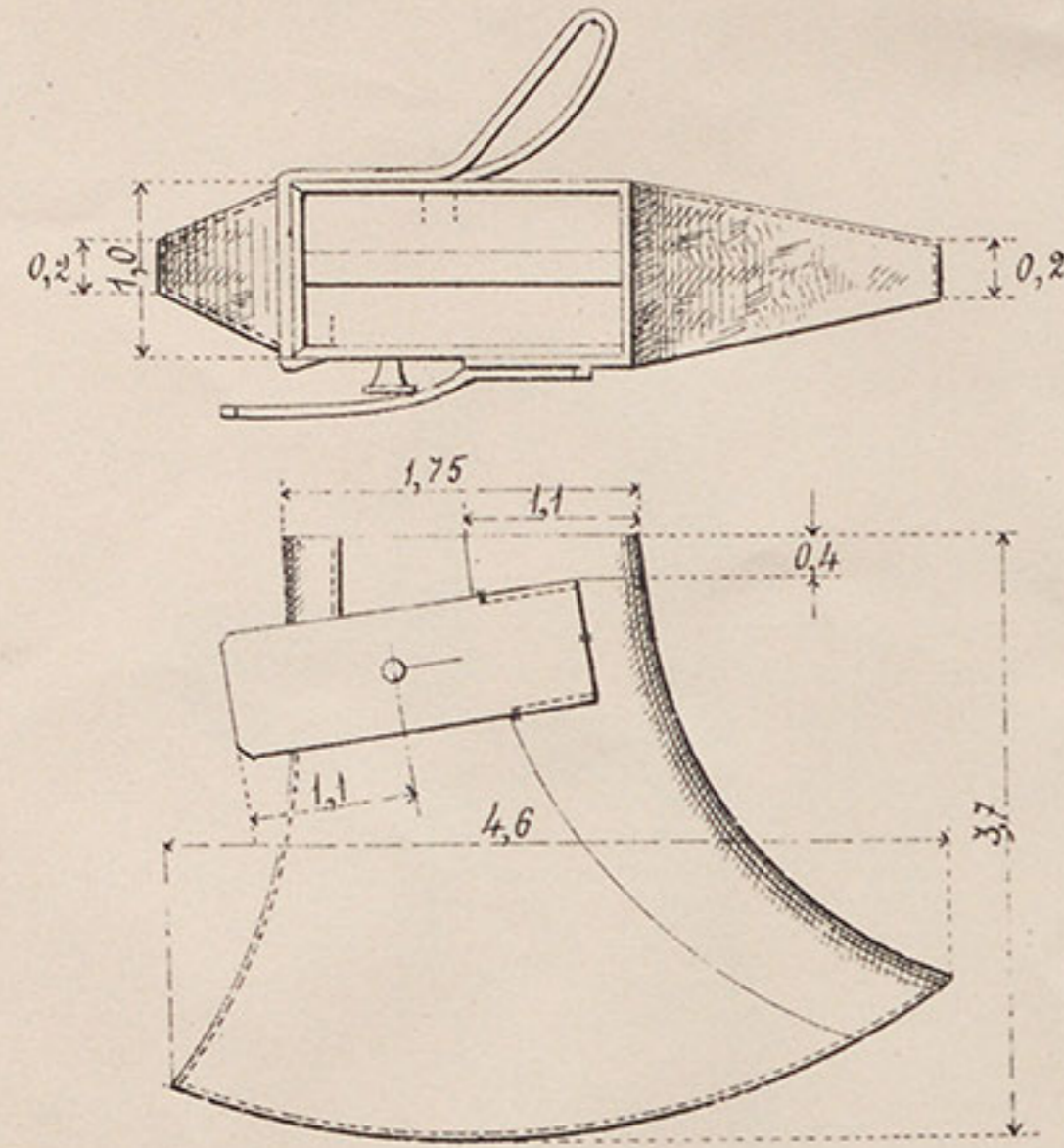
Н. Получахолъ на малый кавалерійскій топоръ.
