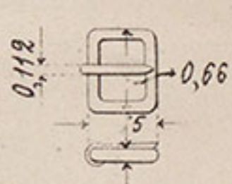
№ 30. Пряжка.
