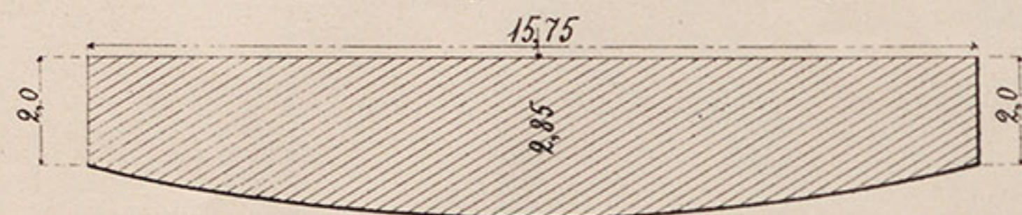
№ 85. Выкройка для задняго соединительнаго ремня.
