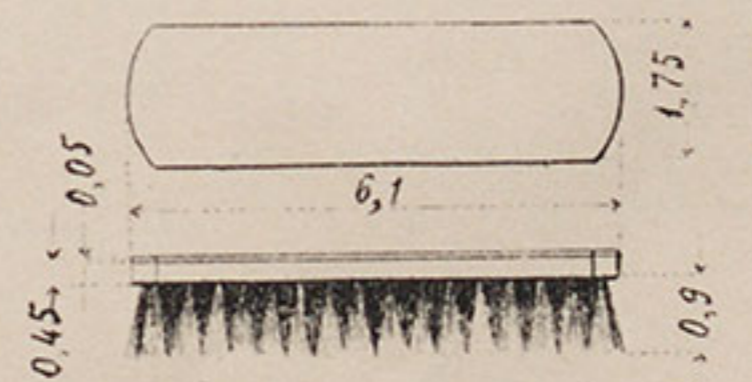
Ж. Щетка платяная или смазная.
