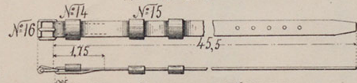
№ 13. Ремень для подбородника.
