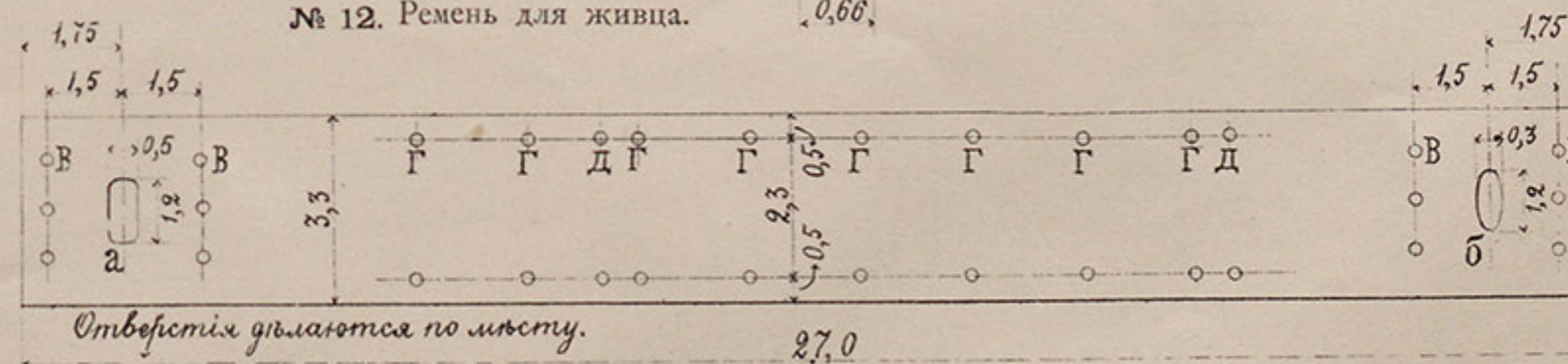
№ 12. Ремень для живца.
