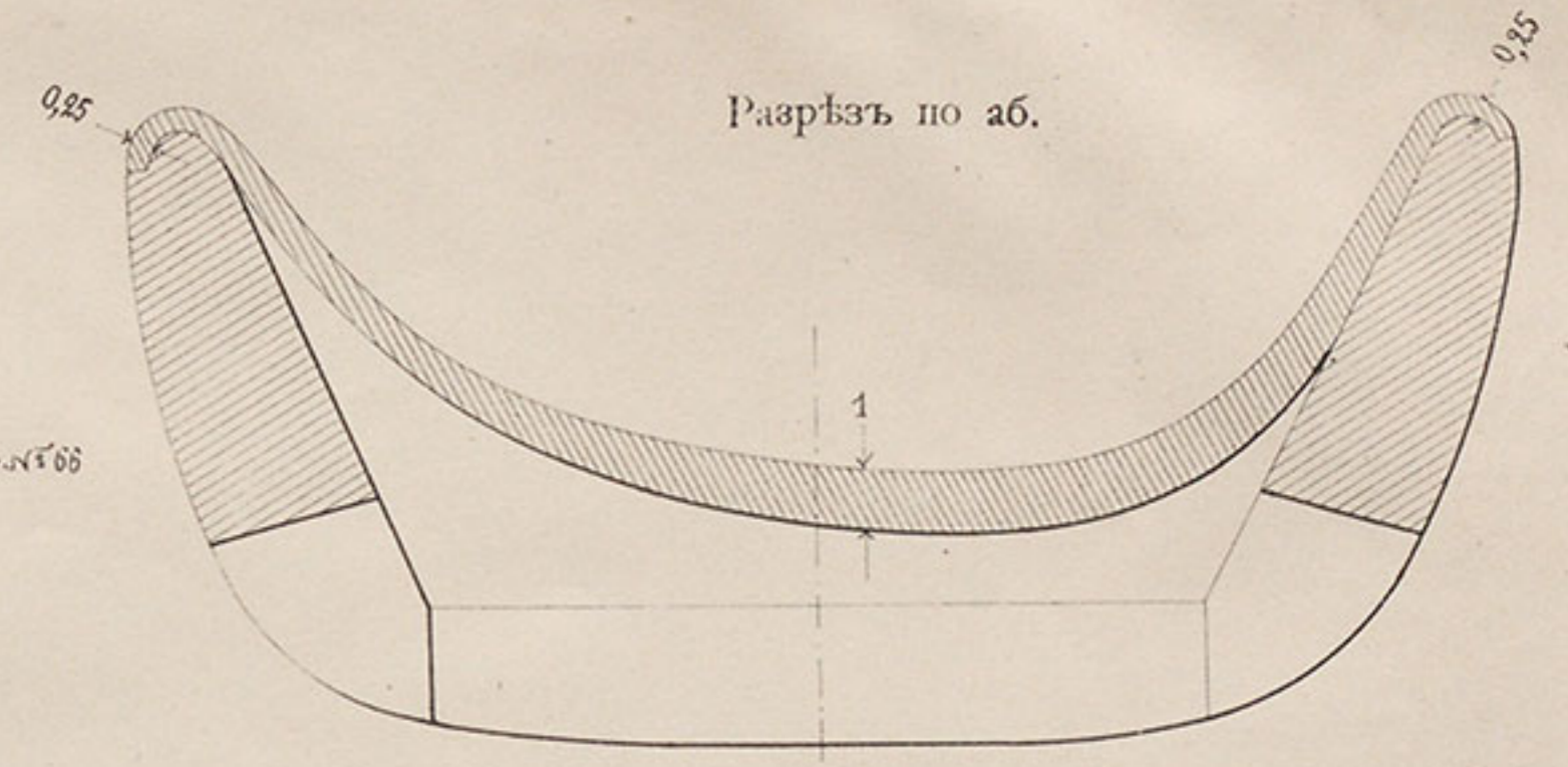
Лекало для сѣченія № I.
