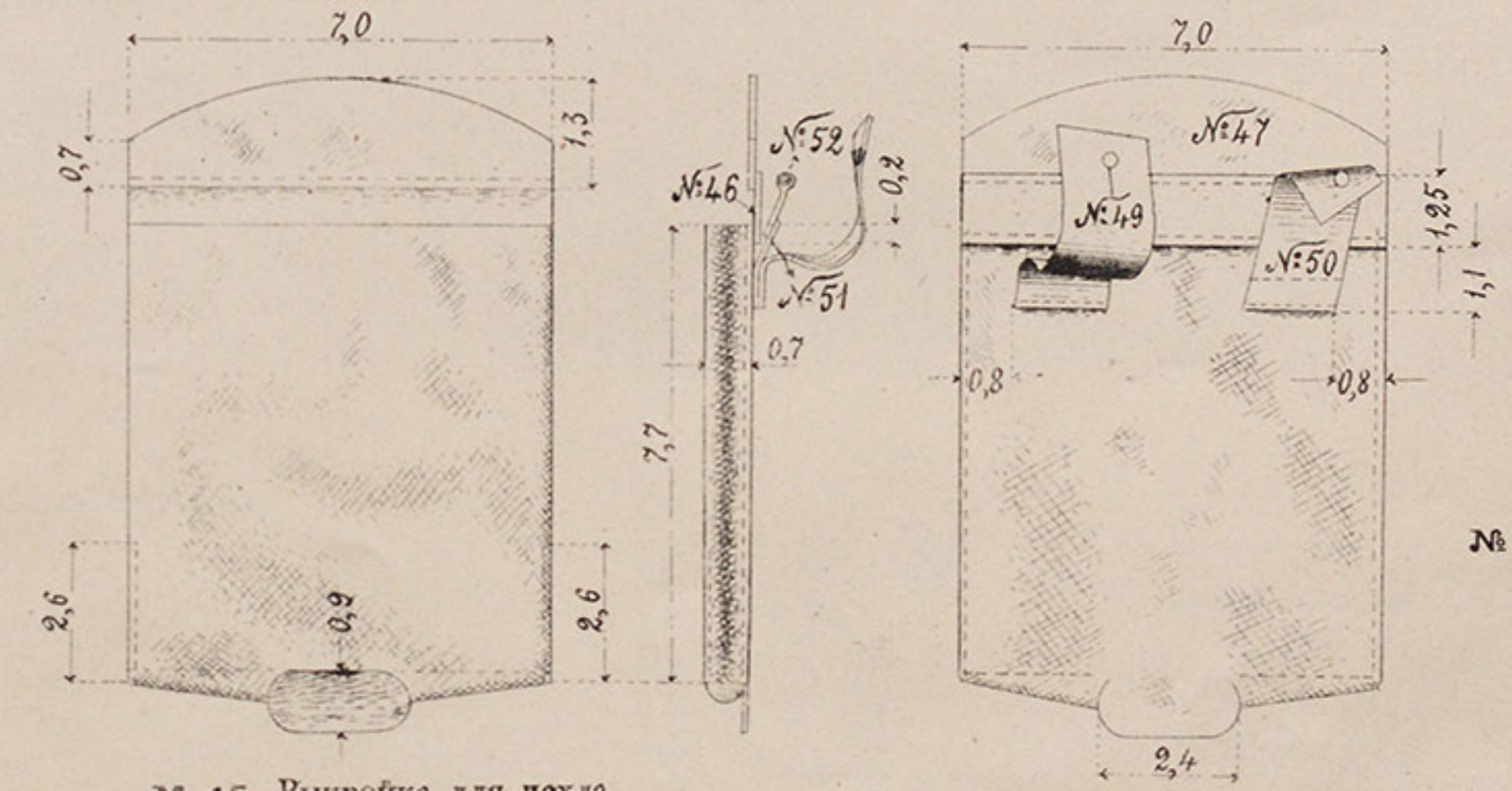
№ 45. Выкройка для чохла.
