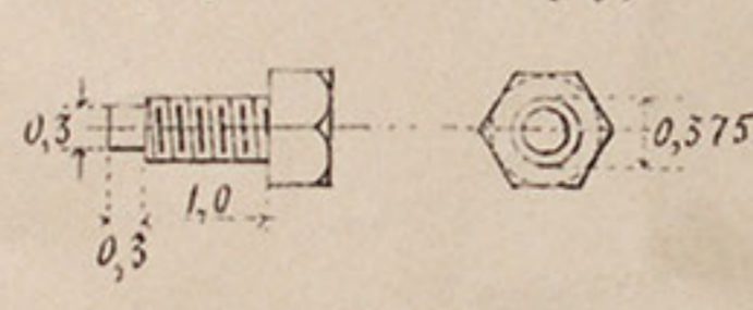
№ 19. Направляющій винтъ. (нарѣзка по Витворту)
