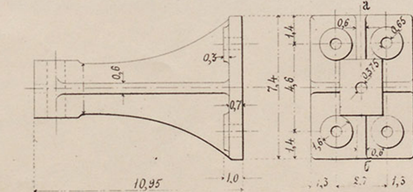
№ 7. Нижній кронштейнъ.
