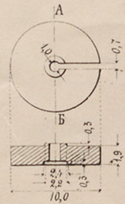
№ 23. Гири.
