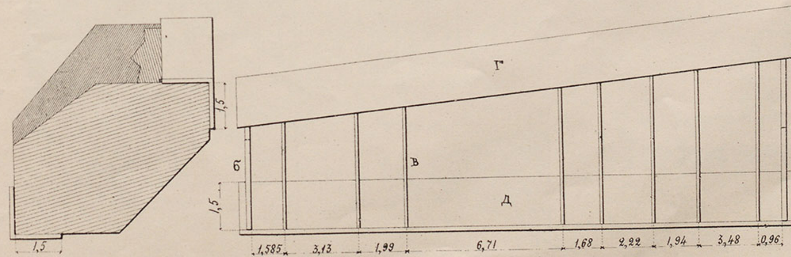
Б. Лекало для отдѣлки лавокъ.
