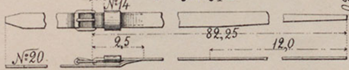
№ 19. Ремень для чумбура.
