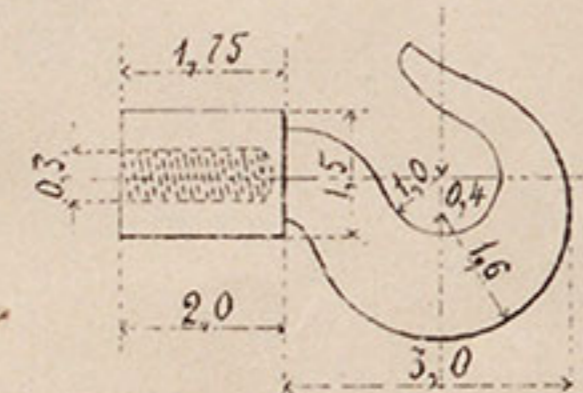
№ 18 Крюкъ къ стержню № 17.
