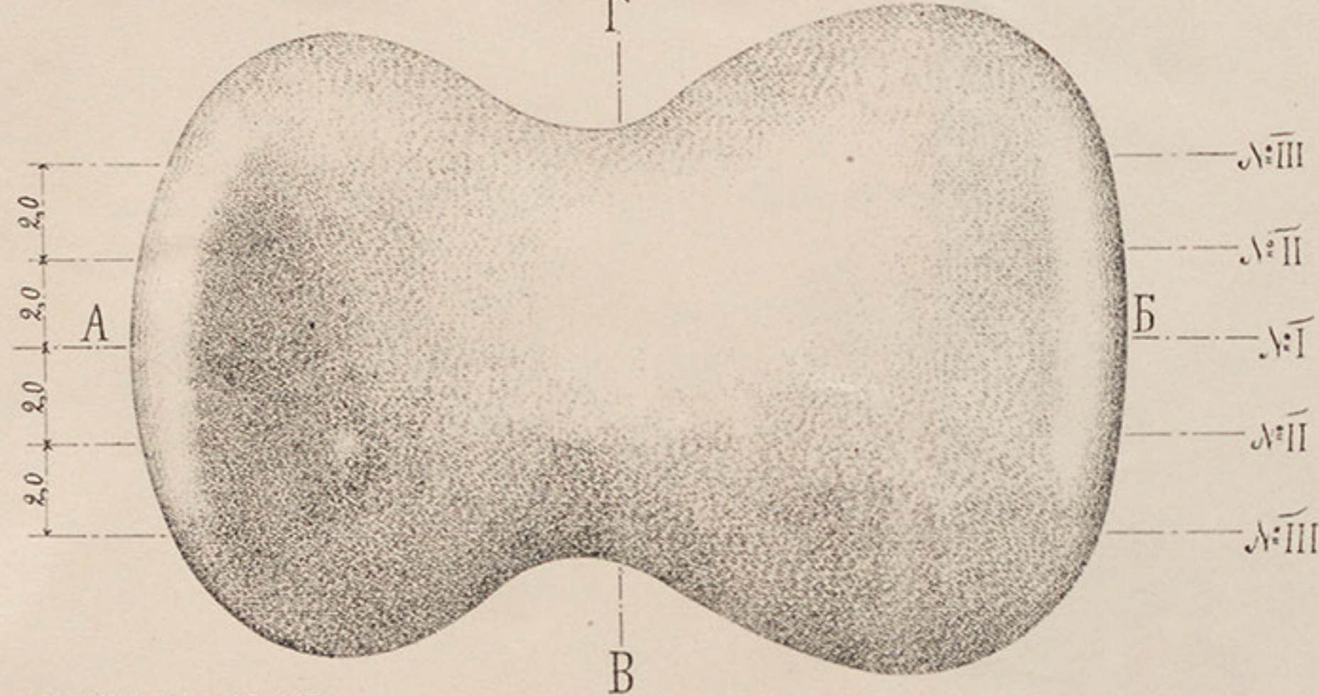
Лекало для сѣченія № III.
