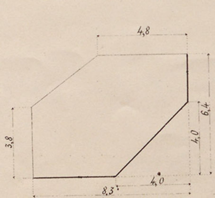
б. Пластика къ лекалу Б.
