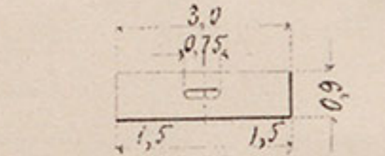
№ 67. Выкройка для мѣшечка.
