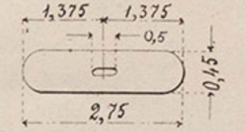
№ 31. Ремешокъ для гайки.
