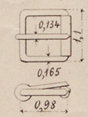
№ 40. Пряжка.
