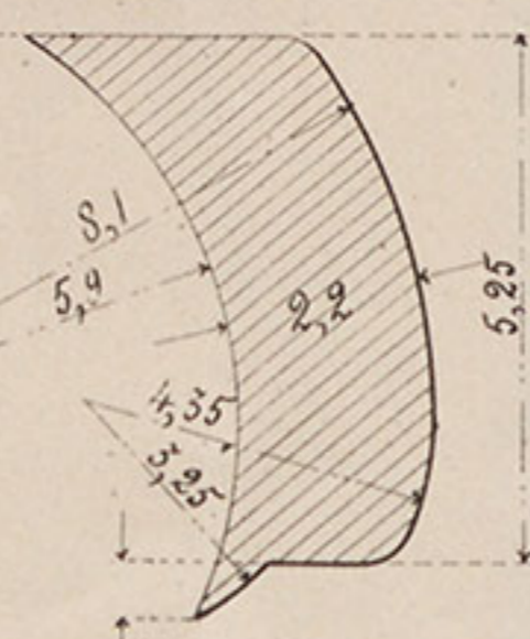
№ 23. Выкройка для клапана.
