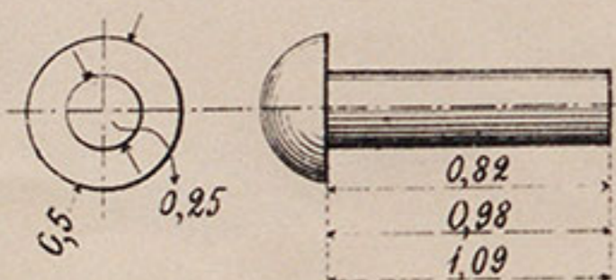
№№ 9, 10 и 11 Заклепки.
