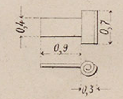
№ 52. Костылекъ.
