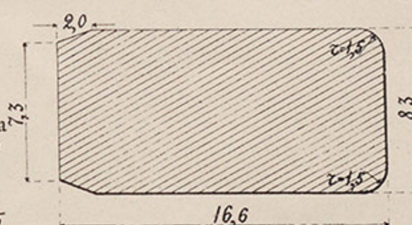
№ 77. Выкройка для крышки.
