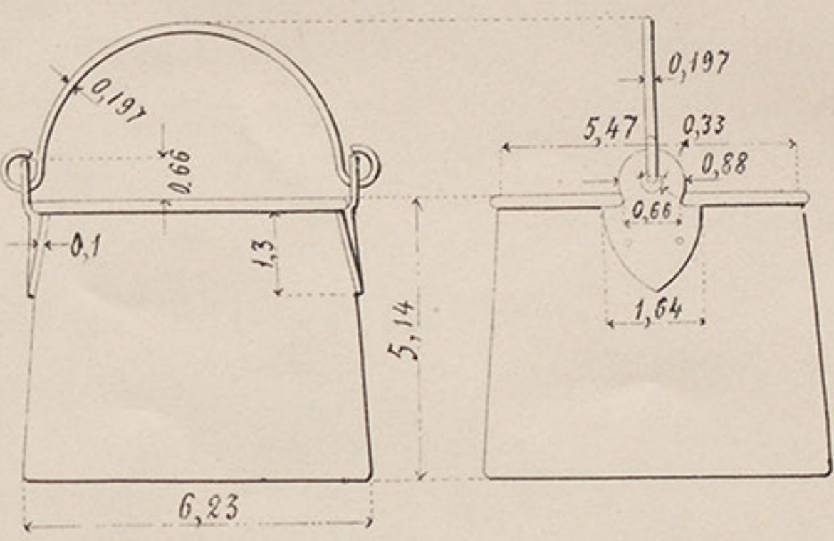
I. Водоносная фляга.
