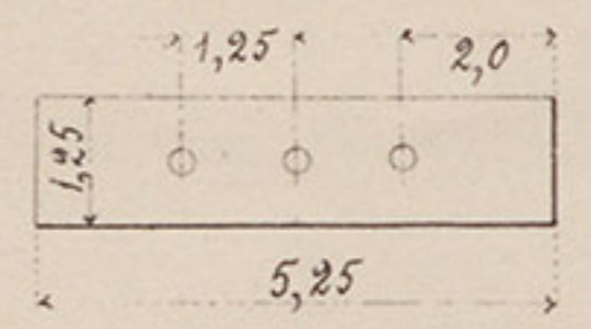
№ 54. Ремешъ для подшивки.
