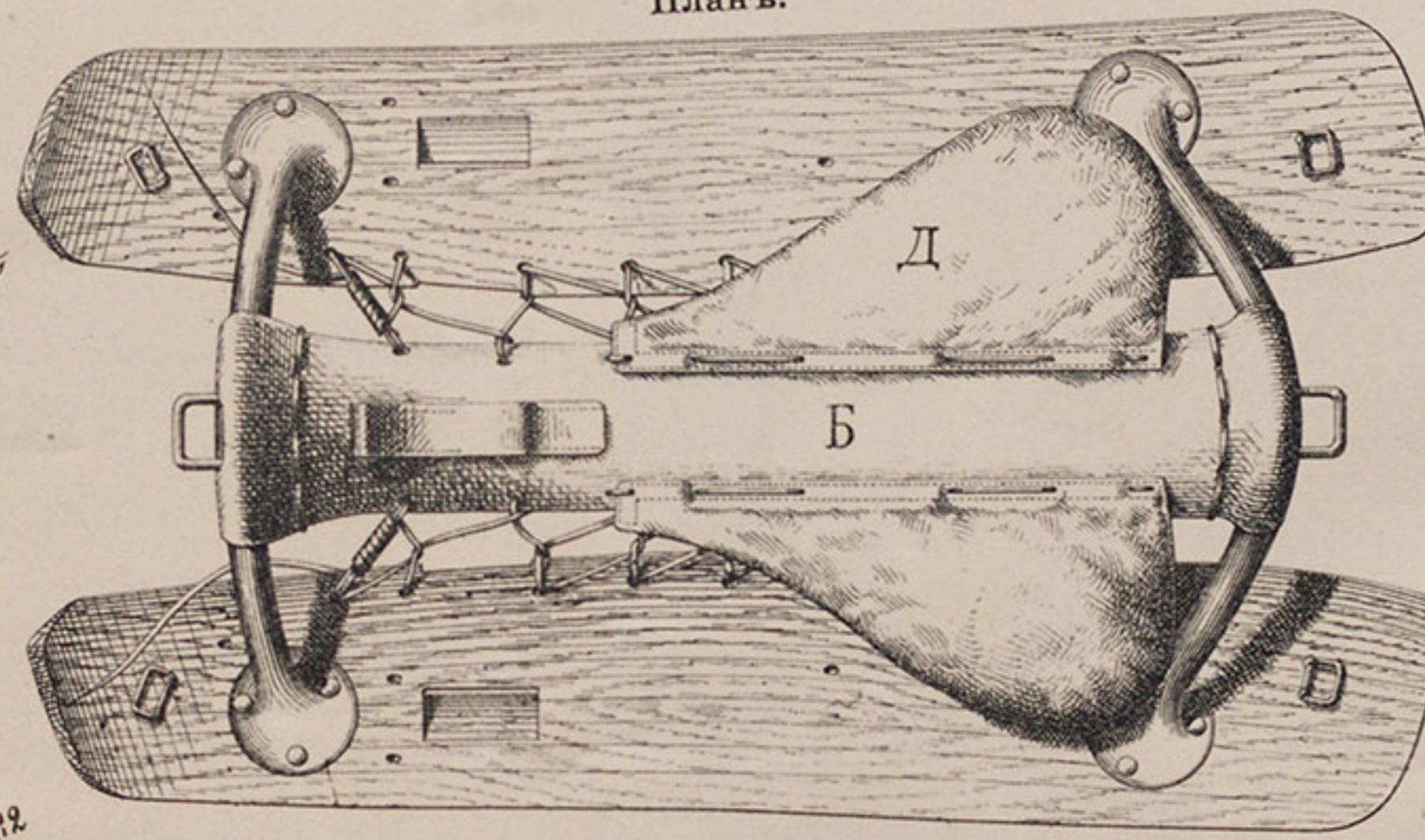
Лапка луки.
