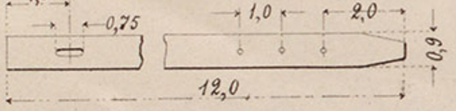
№ 42 Ремень.
