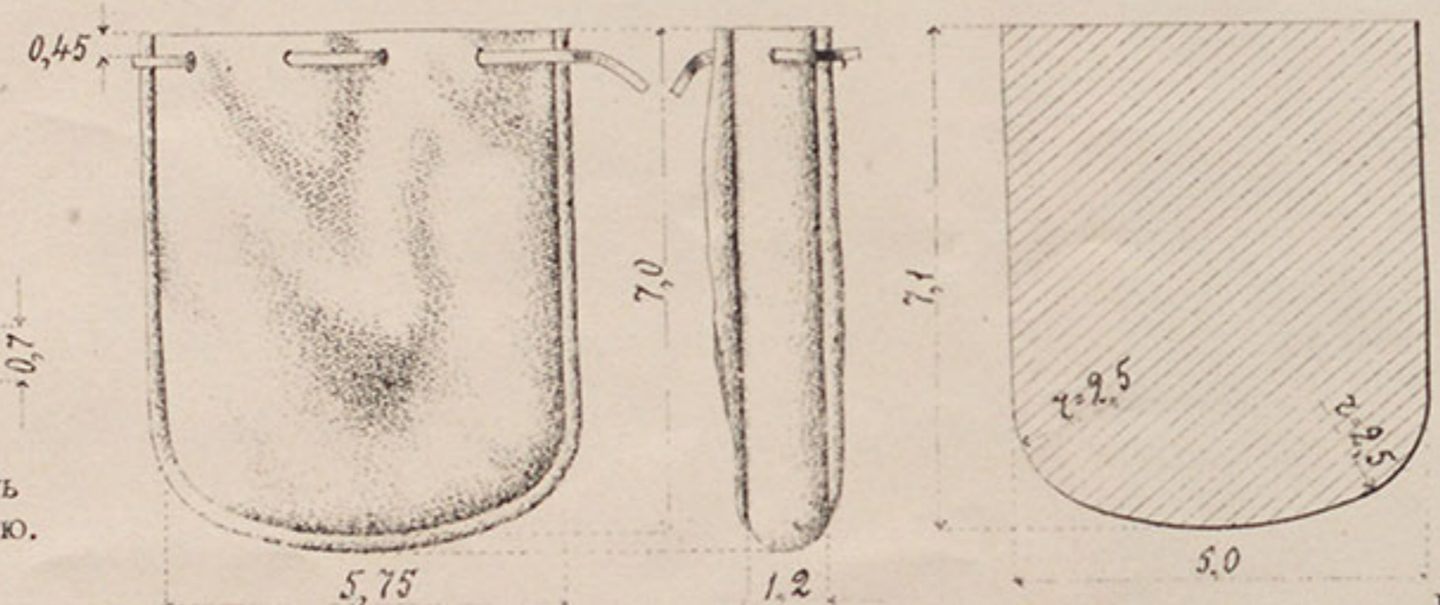
Д. Мѣшечекъ для револьв. прин.
