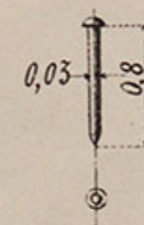
№ 4. Шпилька.
