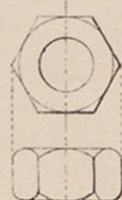
№ 10. Гайка къ болтамъ № 8 и 9.
