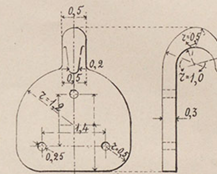
№ 26. Болтикъ къ планкѣ № 25 (нарѣзка по Витворту).
