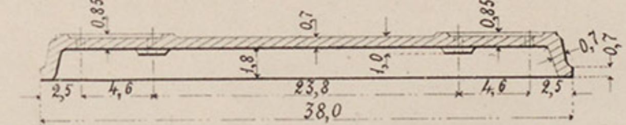
№ 7. Нижній кронштейнъ.
