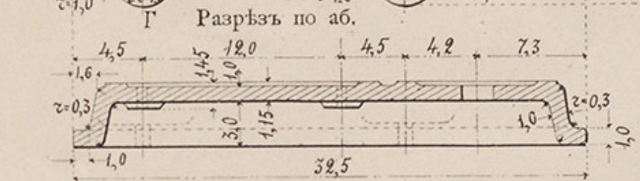
№ 5. Накладная доска.
