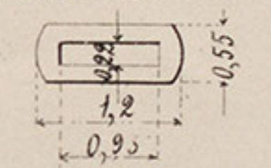
№ 33. Пряжка.
