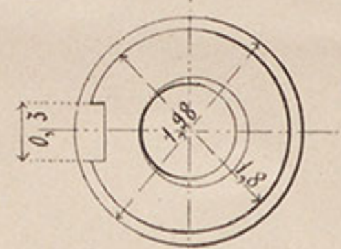
№ 18. Матка къ винту № 11.
