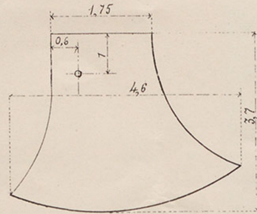
№ 54. Выкройка для доньшка.
