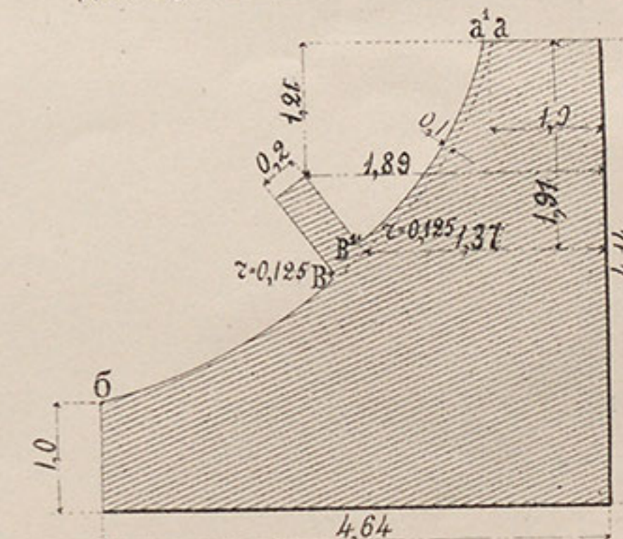
Г. Лекало для повѣрки отверстія для путлища.
