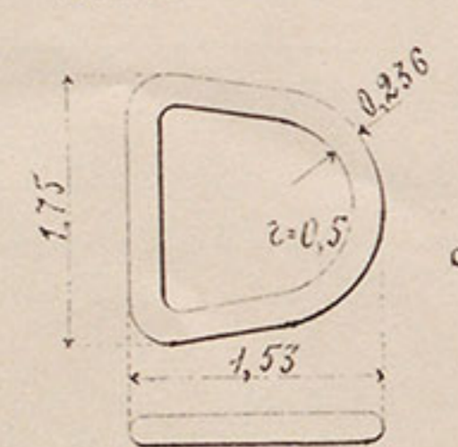
№ 52. Кольцо.
