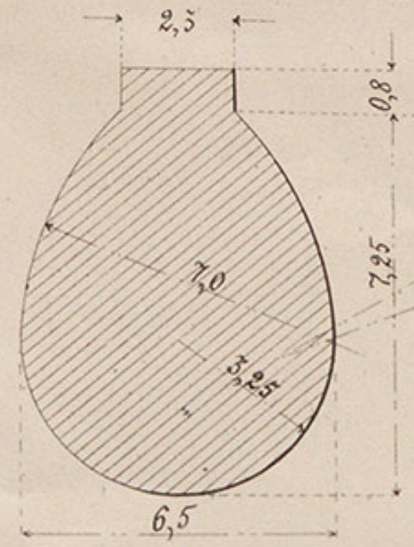
№ 22. Выкройка для чохла.
