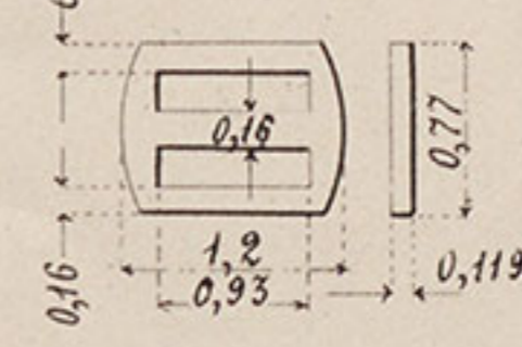
№ 33. Пряжка.
