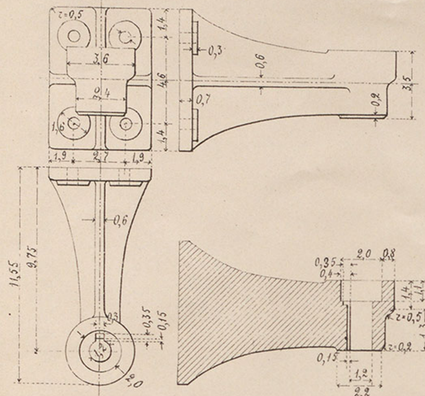
№ 6. Верхній кронштейнъ.
