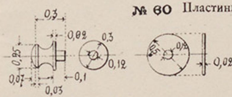
№ 59. Кнопка.
