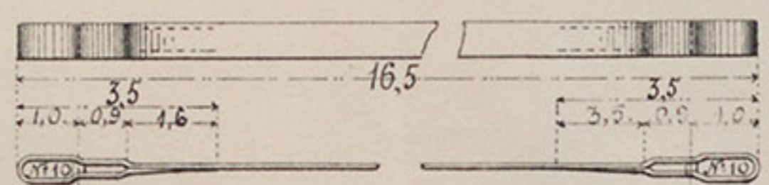
№ 9. Ремень для налобника.
