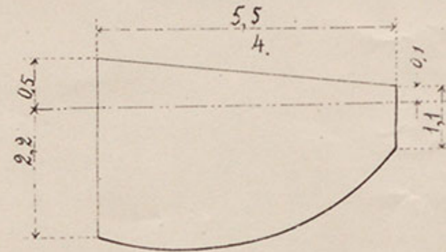
№ 55. Выкройка для крышки.
