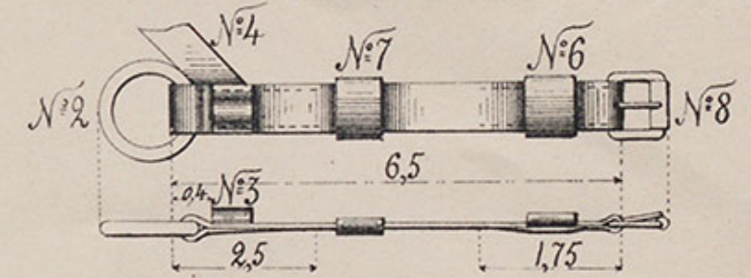
№ 5. Ремень для щечнаго ремня.
