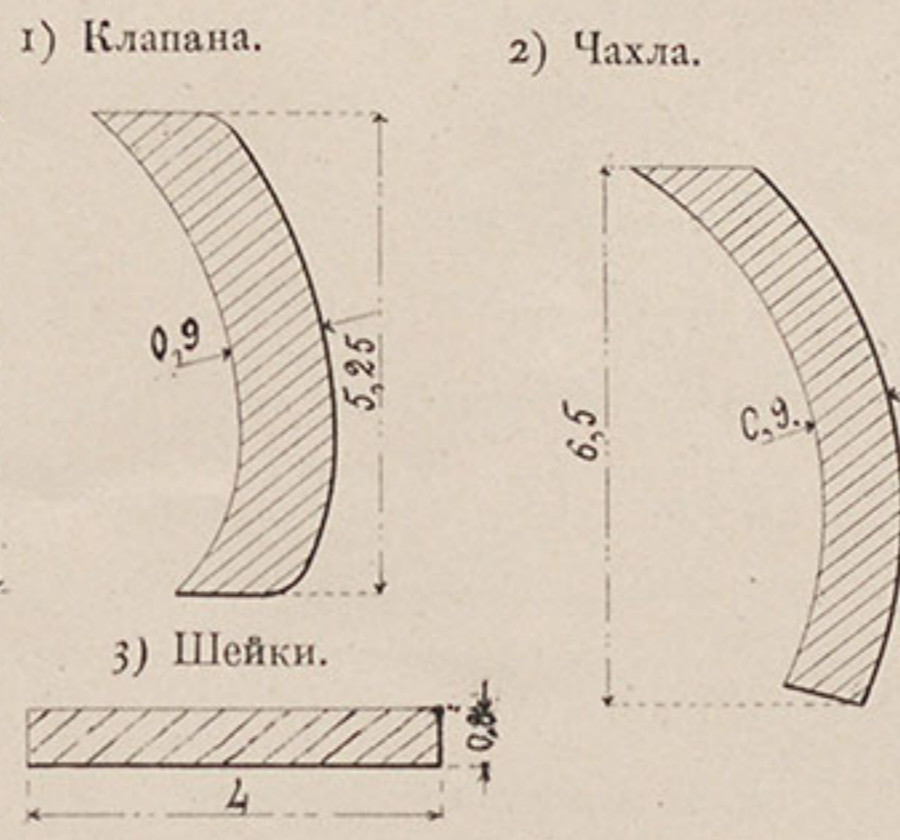
№ 48. Полоска.
