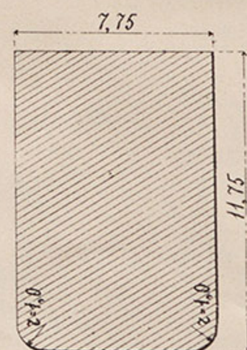
№ 73. Выкройка для задней стѣнки.
