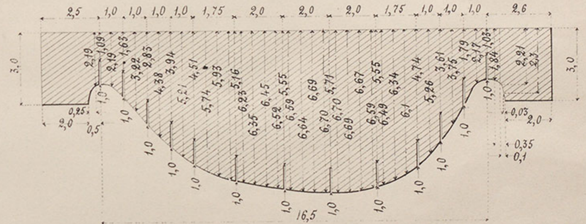
Лекало для сѣченія № II.
