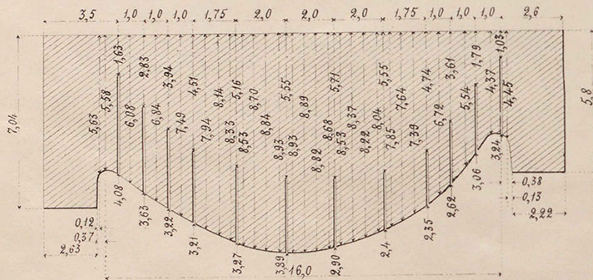
Лекало для сѣченія № III.
