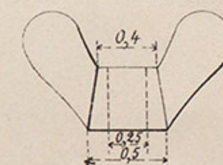
№ 27. Гайка къ болту № 26.
