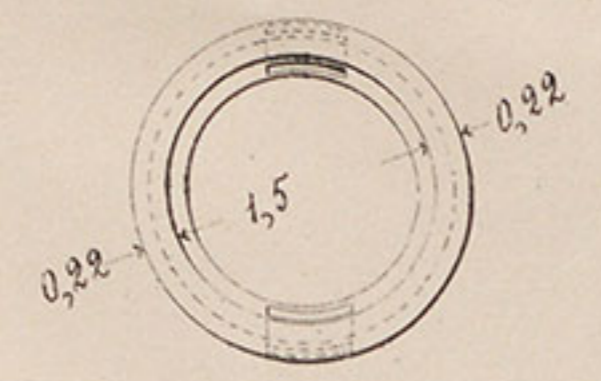
№ 58. Кольцо.
