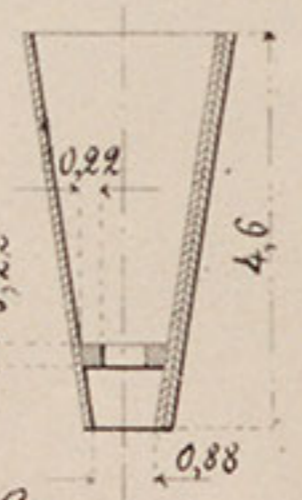
№ 35. Трубка.
