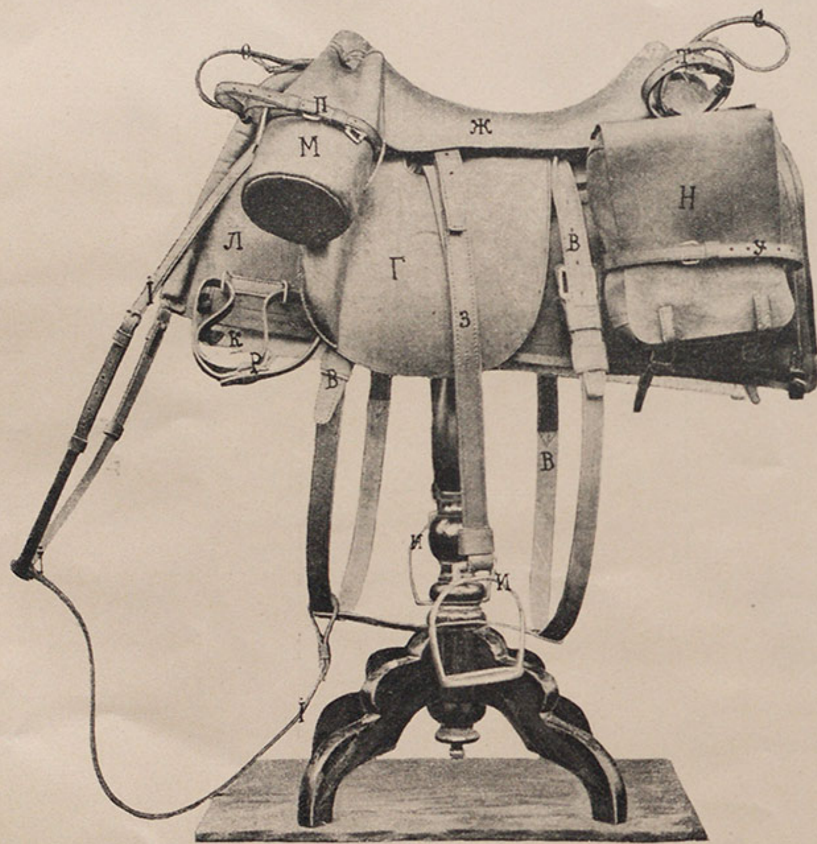
Видъ сбоку.
