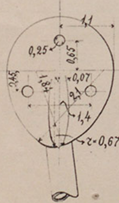
Лапка луки.
