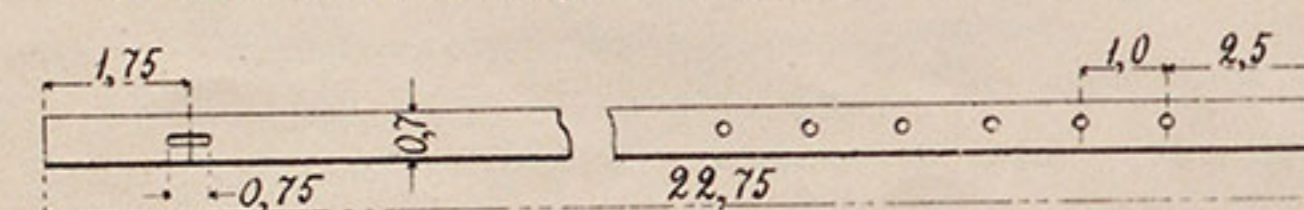
№ 87. Ремень для передняго средняго вьючнаго ремня.
