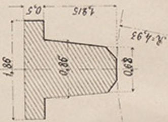
№ 61. Лекало къ станку.
