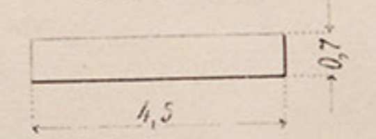
№ 56. Ремешокъ къ соединительному ремню.
