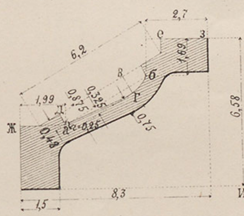
Пластика для сѣченія № 8.
