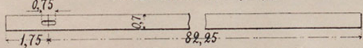
№ 15. Ремешокъ для гайки.
