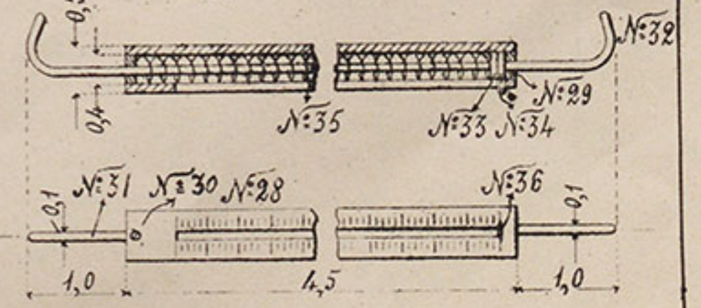
в). Пружинный указатель.
