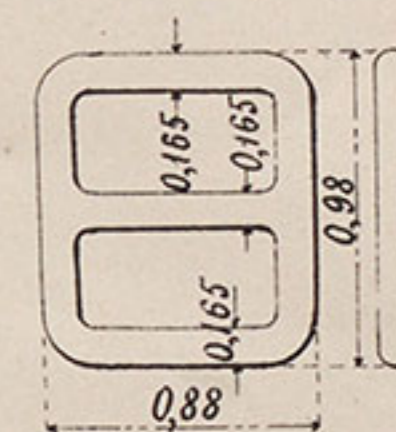
№ 81. Пряжка.
