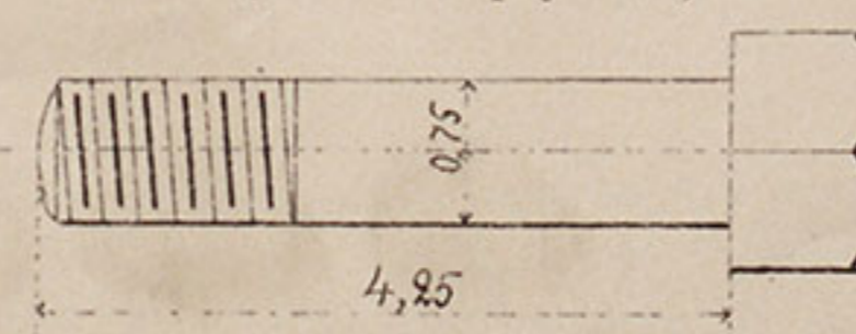
№ 3. Болтъ.
