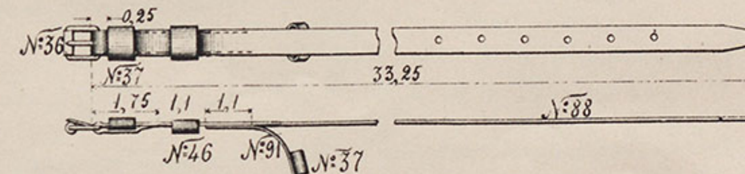
№ 88. Ремень для задняго боковаго вьючнаго ремня.
