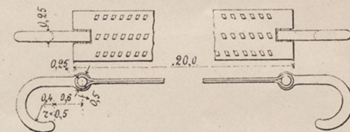
К. Лекало для пригонки луковъ.
