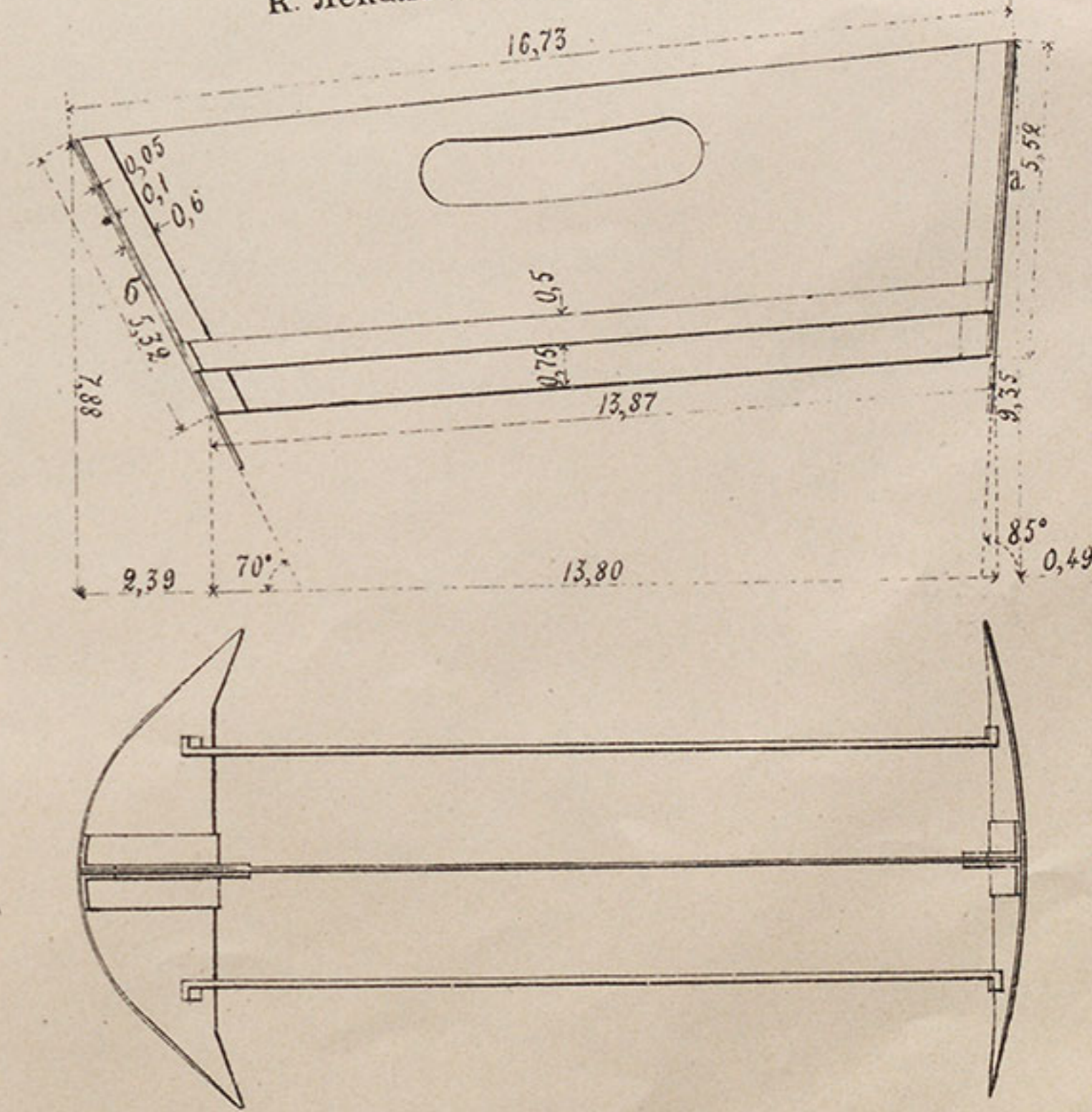
К. Лекало для пригонки луковъ.
