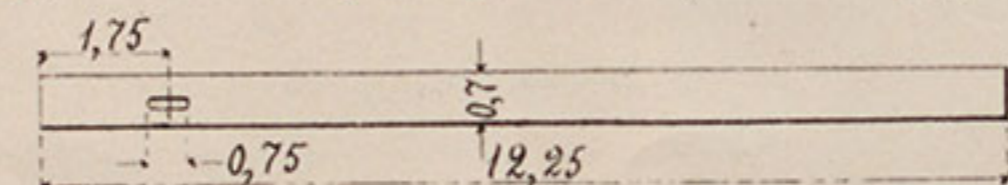
№ 89. Ремень къ переднему боковому вьючному ремню.
