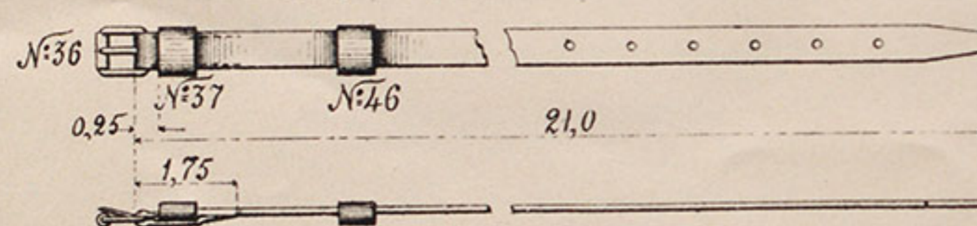
О. Передній средний вьючный ремень.
