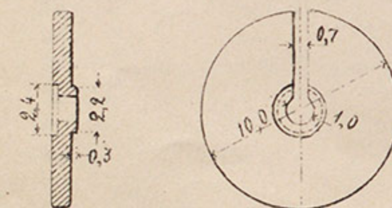
№ 24. Гири.
