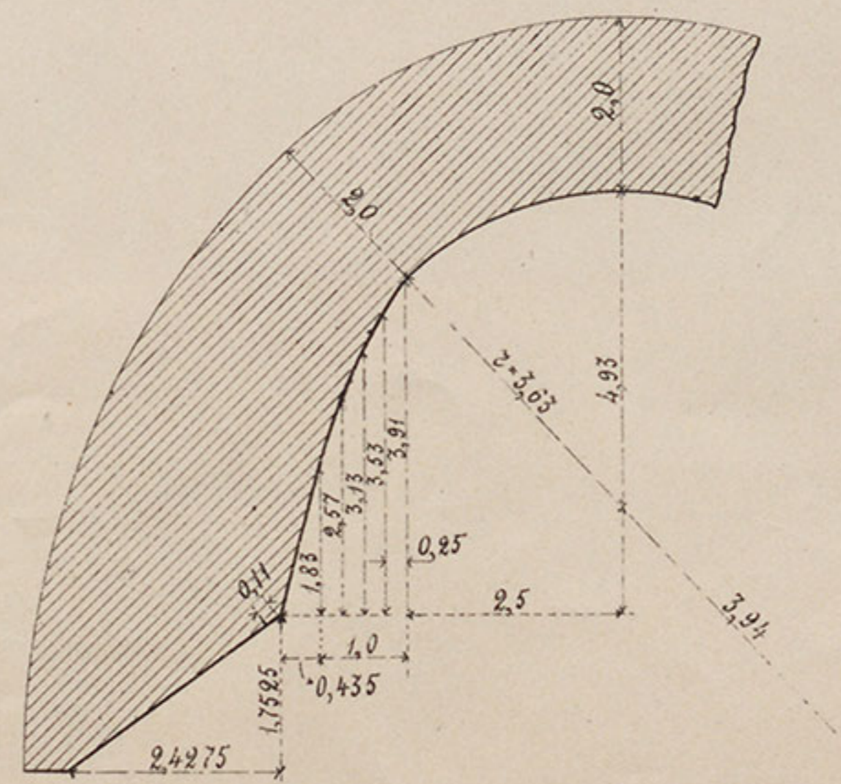
№ 57. Лекало къ станку Ж.
