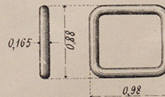
№ 2. Пряжка
