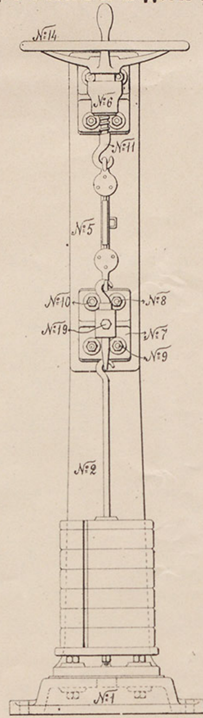
№ 23. Гири.
