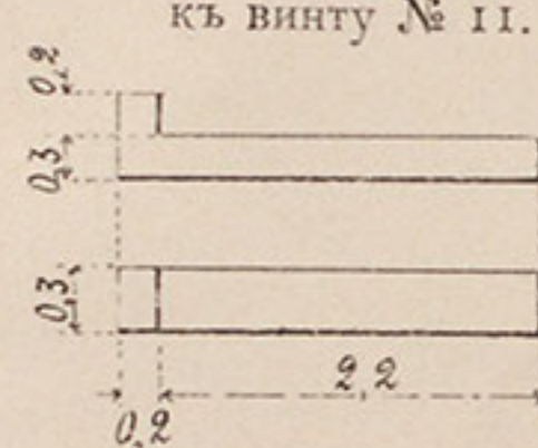
№ 12. Шпонка къ винту № 11.
