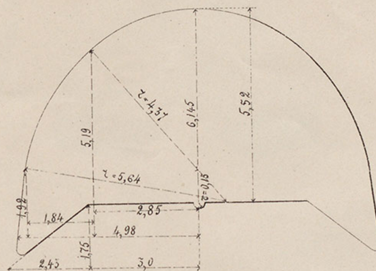
б. Пластина къ лекалу К.
