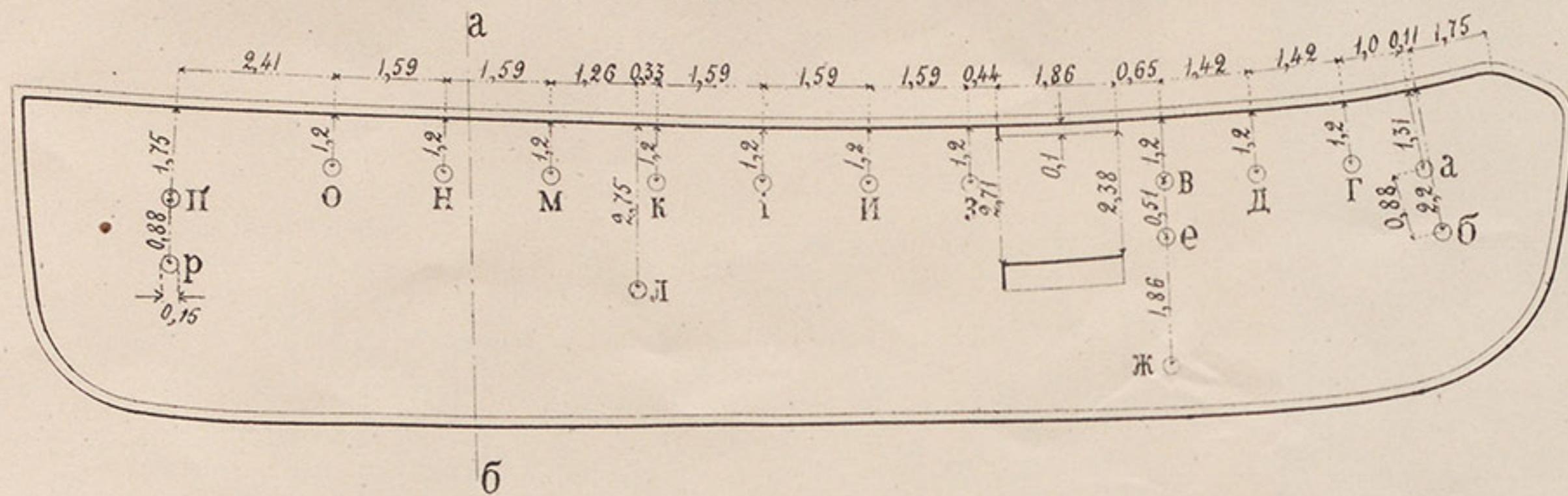
В. Лекало для отверстій въ лавкахъ.
