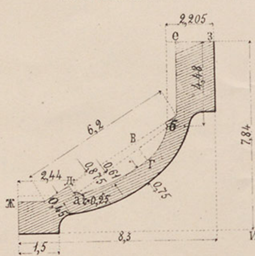
Пластика для сѣченія № 4.
