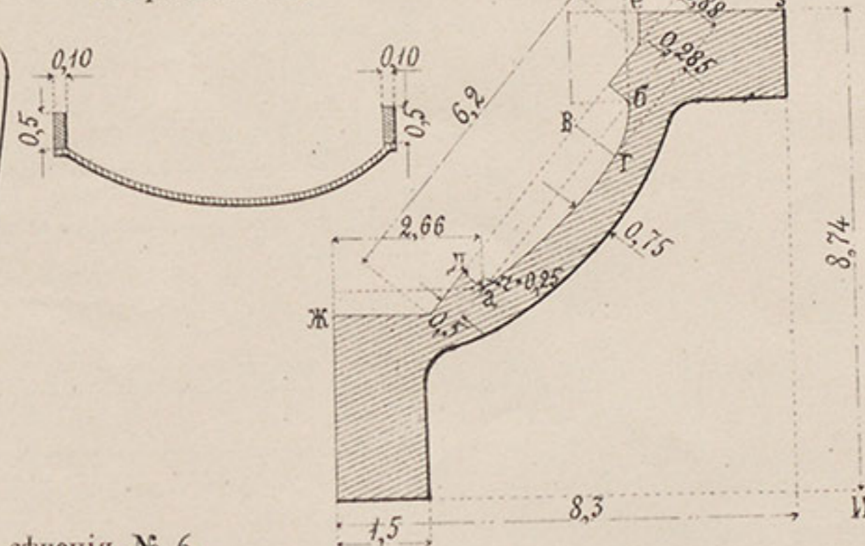
Пластика для сѣченія № 8.
