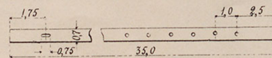
№ 88. Ремень для передняго нижняго вьючнаго ремня.
