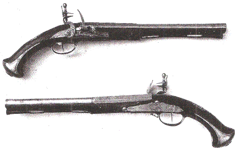
Ett par flintlåspistoler, signerade Nusbaum STOCKHOLM. Total längd 48,5 cm. Pipornas längd 31 cm, slätborrade. Beslag av järn. Kaliber 15 mm. (Livrustkammaren)
