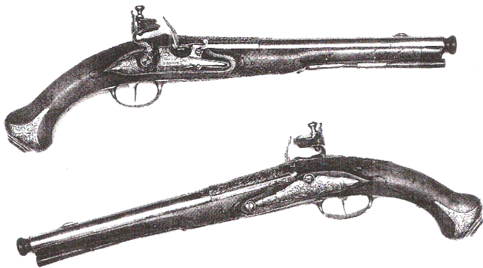
Ett par flintläspistoler, signerade BERG NORKÖPING. Total längd 40 cm. Pipornas längd 25 cm, slätborrade. Järnbeslag med guldpunsad botten. Kaliber 13 mm. (Privat ägo)
