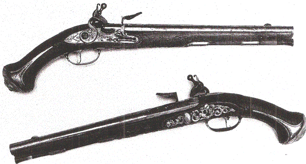
Ett par flintläspistoler, signerade E:WESSMAN STOCKHOLM. Total längd 48 cm. Pipornas längd 32 cm, slätborrade. Beslag av järn. Kaliber 15 mm. (Privat ägo)
