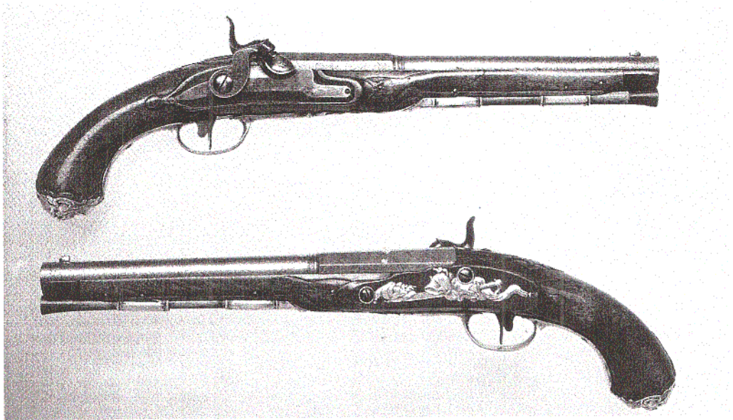
Ett par slaglåspistoler, ändrade från flintlås, signerade A.GERHARDT STOCKHOLM. Total längd 40 cm. Pipornas längd 26 cm, slätborrade. Å piporna Fredrik I:s krönta namnchiffer FRS i guld. Beslag av silver. Kaliber 15 mm. (Privat ägo)
