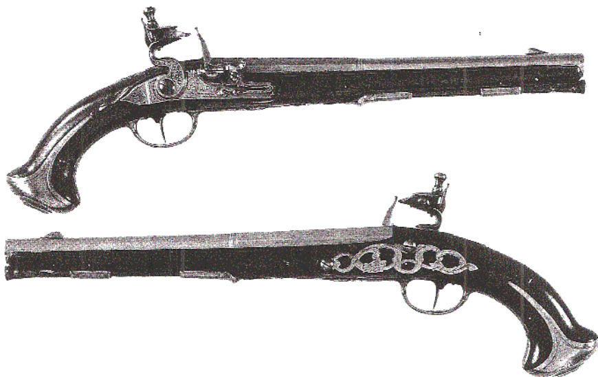
Ett par flintlåspistoler, signerade Fallgren Jönköping. Total längd 47 cm. Pipornas längd 30,5 cm, släthorrade. Beslag av järn. Kaliber 15 mm. (Livrustkammaren)
