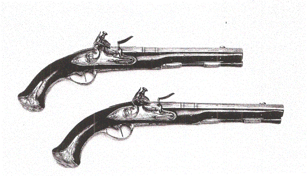
Ett par flintläspistoler, signerade MELLBERG. Total längd 39 cm. Pipornas längd 24 cm, släitborrade. Beslag av järn. Kaliber 15 mm. (Privat ägo)
