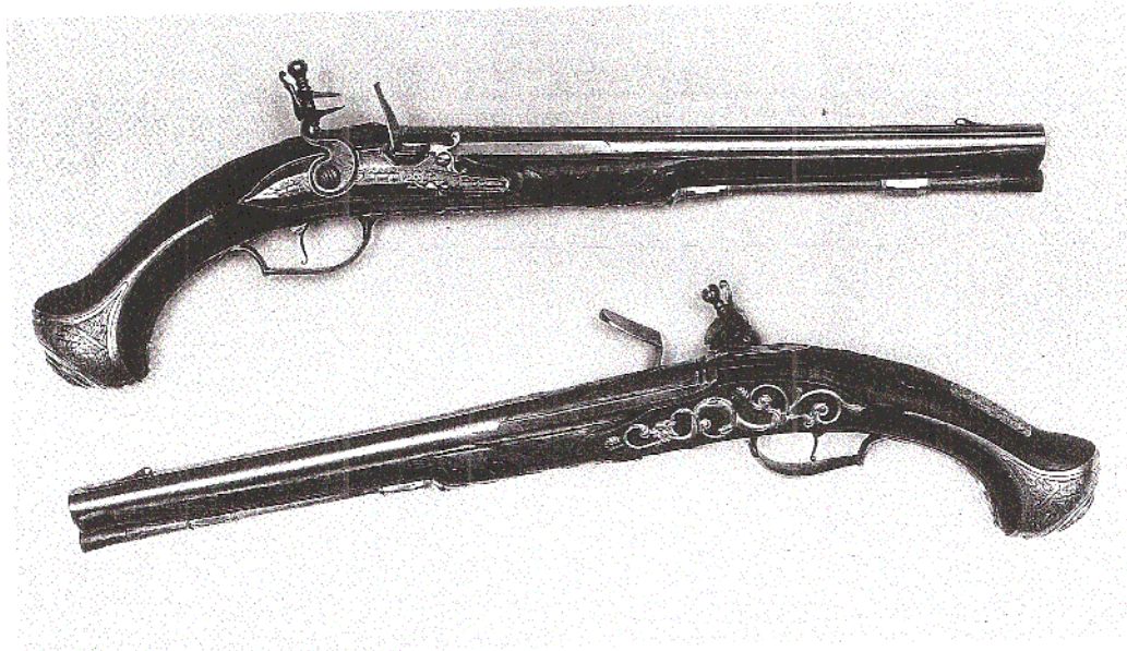
Ett par flintlåspistoler, signerade L:BLEKBERG. Total längd 50,5 cm. Pipornas längd 33 cm, slätborrade. De bär inskriptionen "JönKiöping". Beslag av mässing. Kaliber 15 mm. (Privat ägo)
