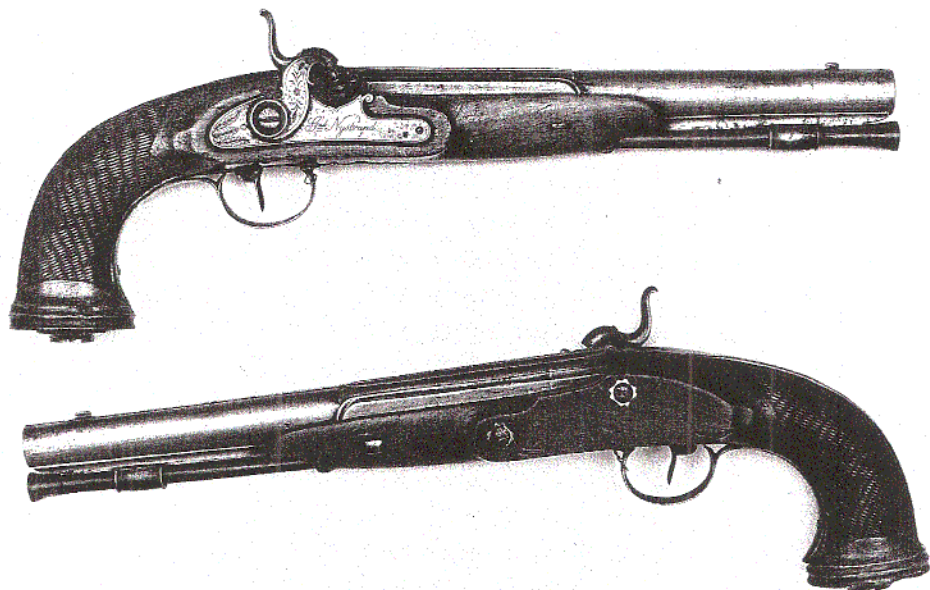
Ett par slaglåspistoler, signerade G nd Nystrand. Total längd 38,5 cm. Pipornas längd 26 cm, räfflade. Beslag av järn. Kaliber 16 mm. (Privat ägo)
