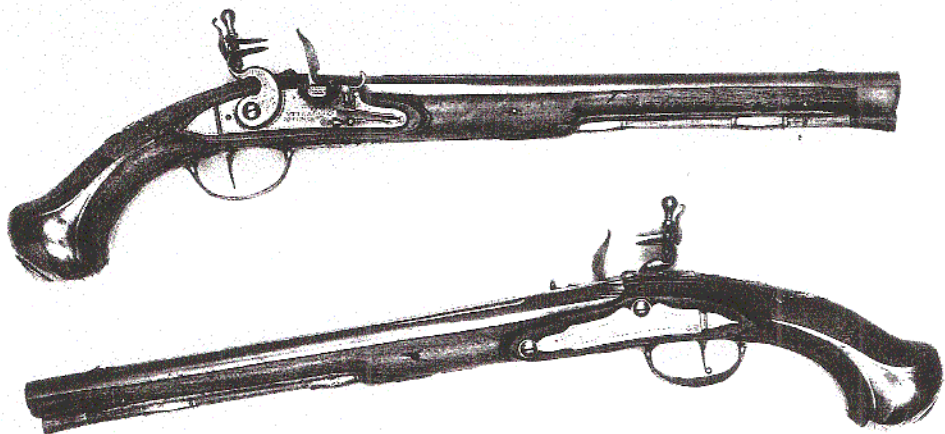
Ett par flintlåspistoler, signerade UTTERBERG NORKIÖPING. Total längd 54 cm. Pipornas längd 36 cm, slätborrade. De är signerade FELIX MEIER IN WIENN. Beslag i järn. Kaliber 16 mm. (Privat ägo)
