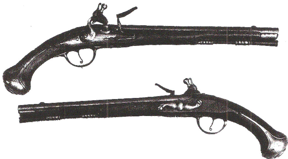
Ett par flintlåspistoler, signerade TESCHNER STOKHOLM. Total längd 45,5 cm. Pipornas längd 31 cm, slätborrade. Beslag av järn. Kaliber 14 mm. (Privat ägo)
