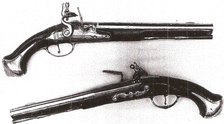
Ett par flintlåspistoler, signerade S:ÅLANDER. Total längd 44 cm. Pipornas längd 28 cm, slätborrade. Beslag av mässing. Kaliber 17 mm. (Privat ägo)
