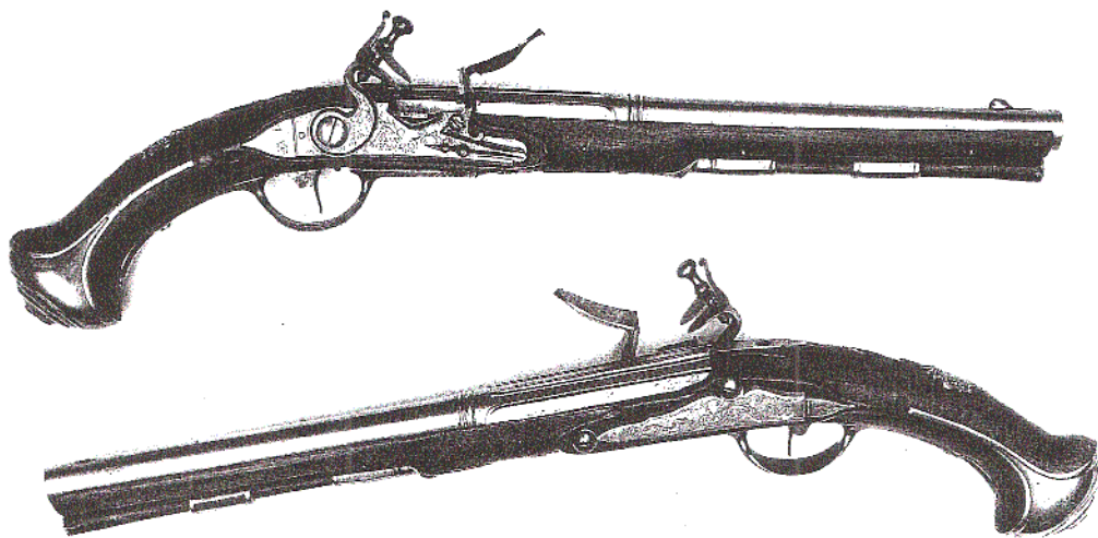
Ett par flintlåspistoler, signerade D BARS STOCKHOLM. Total längd 48 cm. Pipornas längd 31,5 cm, slätborrade. Beslag av järn. Kaliber 14 mm. (Privat ägo)
