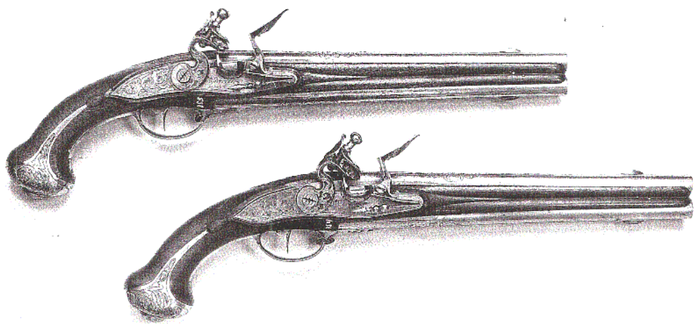
Ett par flintlåspistoler, signerade M:GIÖTTER. Total längd 49 cm. Pipornas längd 30 cm, slätborrade. Förgyllda mässingsbeslag. Kaliber 9 mm. (Privat ägo)
