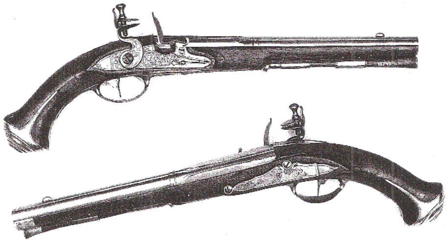
Ett par flintlåspistoler, signerade FRENBERG STOCKHOLM. Total längd 43,5 cm. Pipornas längd 27,5 cm, slätborrade. Beslag av järn. Kaliber 16 mm. (Skokloster)
