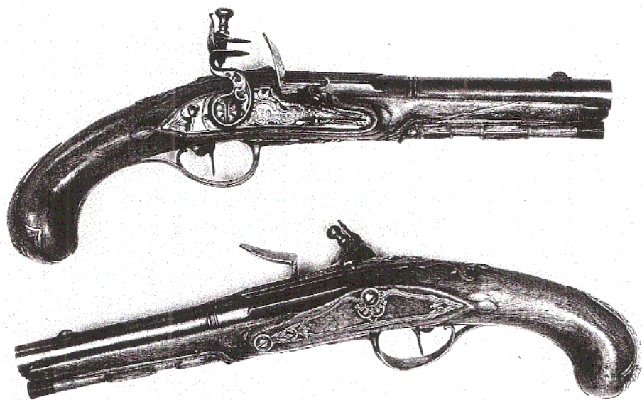
Ett par flintlåspistoler, signerade H:DOMNERUS. Total längd 33 cm. Pipornas längd 18 cm, slätborrade. Beslag av järn. Kaliber 14 mm. (Privat ägo)
