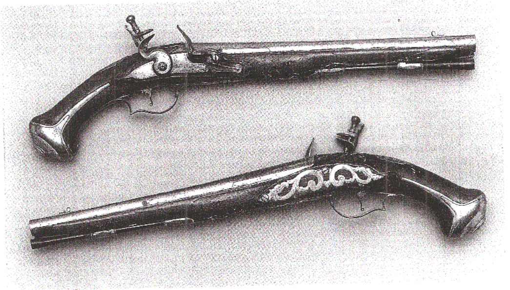
Ett par flintlåspistoler, signerade J:RUBERG. Total längd 50 cm. Pipornas längd 32 cm, slätborrade. Beslag av järn. Kaliber 15 mm. (Privat ägo)
