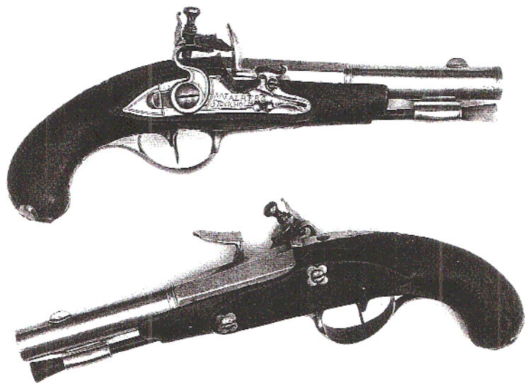
Ett par flintlåspistoler, signerade WÅLBERG STOCKHOLM. Total längd 25 cm. Pipornas längd 14 cm, slätborrade. Beslag av järn. Kaliber 12 mm. (Privat ägo)
