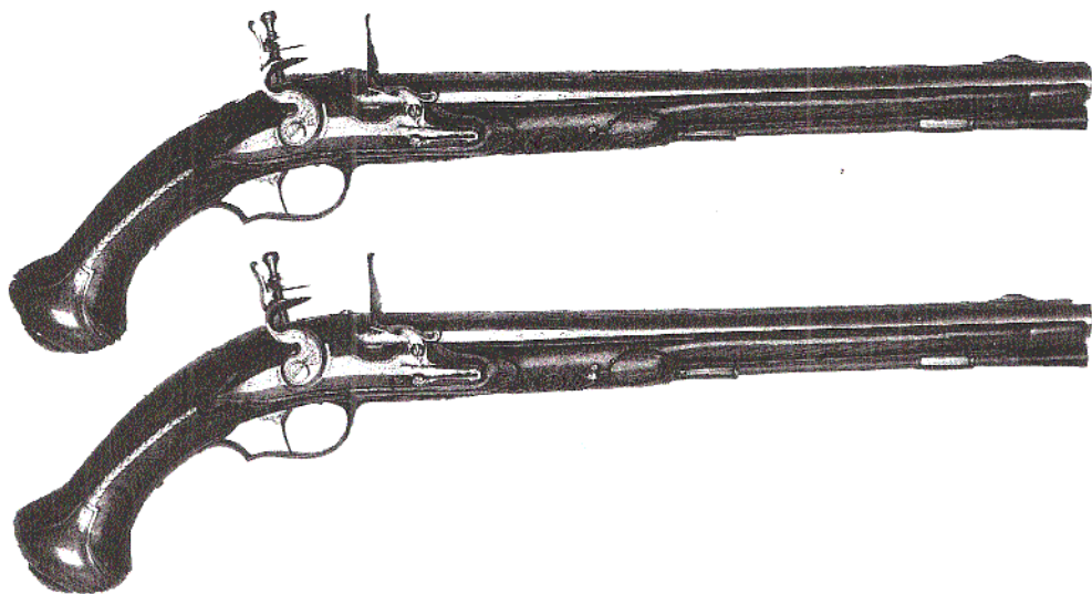
Ett par flintlåspistoler, signerade B:MÅRD. Total längd 53 cm. Pipornas längd 35,5 cm, slätborrade. Beslag av mässing. Kaliber 15 mm. (Privat ägo)
