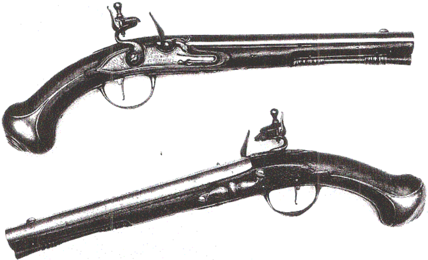
Ett par flintläspistoler, signerade STARBUS STOKHOLM. Total längd 45 cm. Pipornas längd 27,5 cm - en slätborrad, en räfflad. Beslag av järn. Kaliber 16 mm resp. 17 mm. (Privat ägo)
