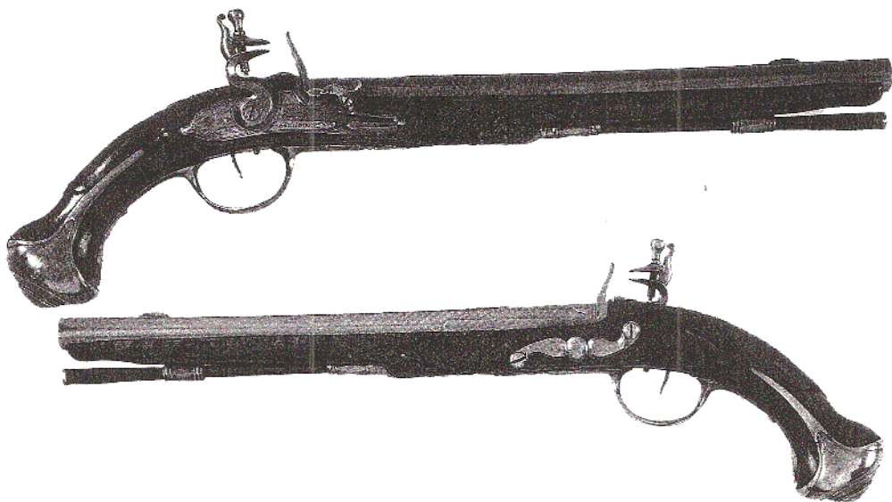
Ett par flintlåspistoler, signerade O:BERGGREN JÖNKIÖPING. Total längd 52,5 cm. Pipornas längd 35 cm, släiborrade. Beslag av mässing. Kaliber 16 mm. (Livrustkammaren)
