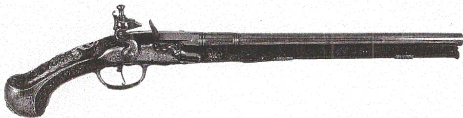
Ett par flintlåspistoler, signerade Peeter Froomen. Total längd 53,5 cm. Pipornas längd 36,5 cm, slätborrade. Beslag av järn. Kaliber 13 mm. (Livrustkammaren)
