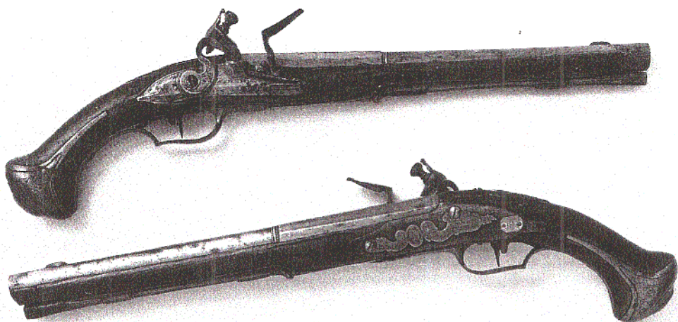
Ett par flintlåspistoler, signerade A:FRENBORG. Total längd 50 cm. Pipornas längd 33 cm, slätborrade. Beslag av mässing. Kaliber 15 mm. (Privat ägo)
