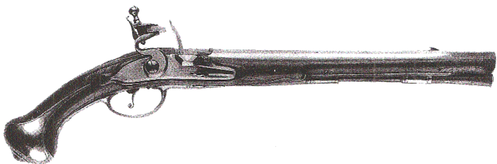
Flintlåspistol, signerad BENGTLILLIA JÖNKÖPING. Total längd 52 cm. Pipans längd 34,5 cm, slätborrad. Beslag av mässing. Kaliber 17 mm. (Armémuseum)
