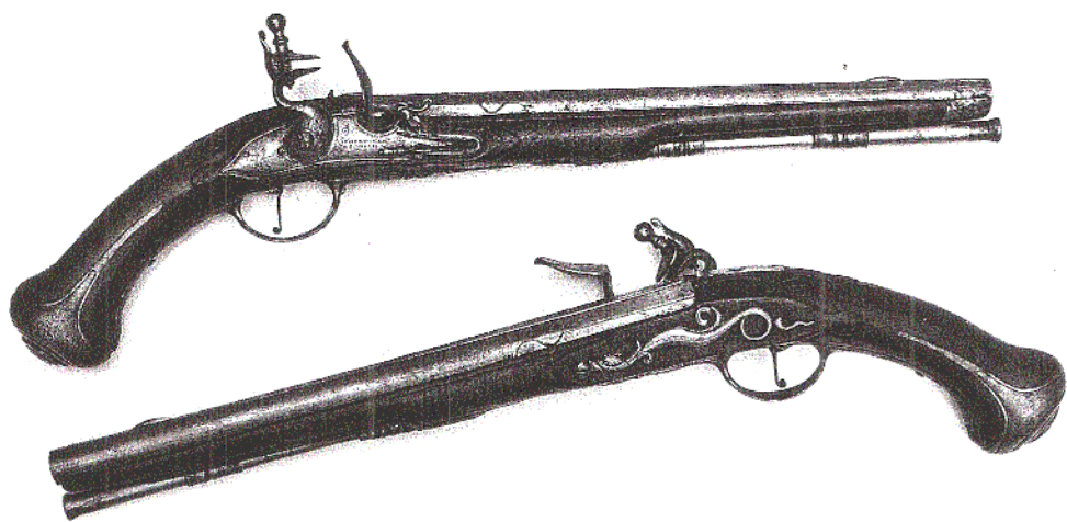
Ett par flintlåspistoler, signerade SCHERTIGER STOCKHOLM. Total längd 50,5 cm. Pipornas längd 33,5 cm, slätborrade. De bär texten LAZARINO COMIAZZO. Beslag av järn. Kaliber 15 mm. (Privat ägo)
