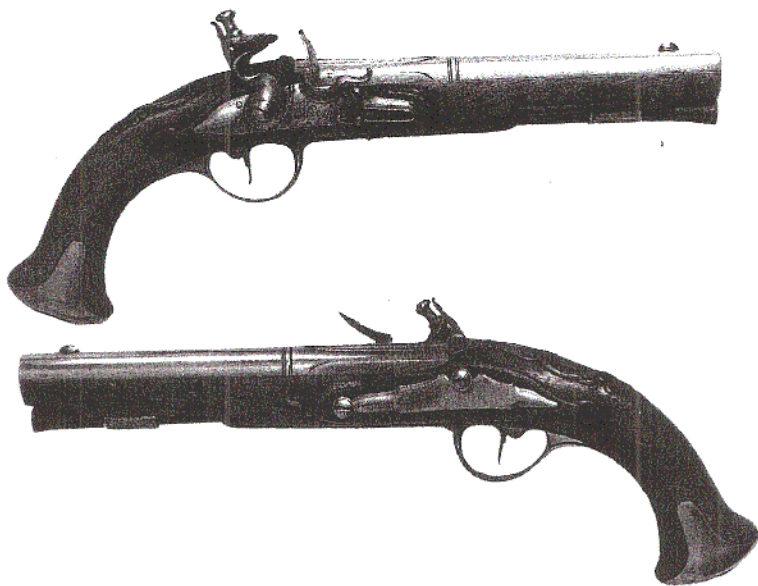
Ett par flintlåspistoler, den ena signerad Gezelius, den andra Söderhamn. Total längd 28,5 cm. Pipornas längd 16,5 cm, slätborrade. Beslag av järn. Kaliber 12 mm. (Kulturen)
