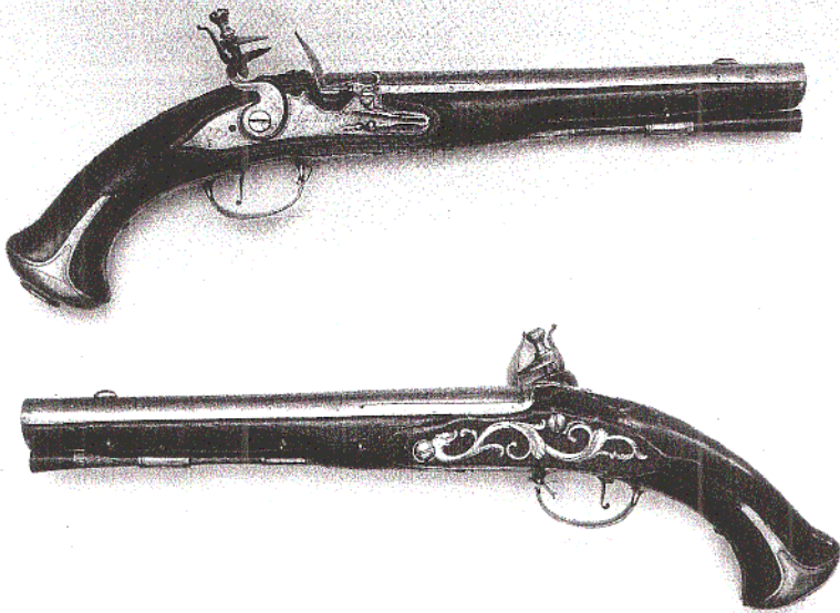
Ett par flintlåspistoler, signerade JOHANN SCHIEL. Total längd 40 cm. Pipornas längd 24,5 cm, slätborrade. Beslag av mässing. Kaliber 15 mm. (Privat ägo)
