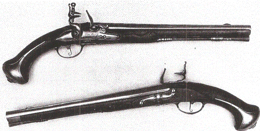
Ett par flintlåspistoler, signerade DAVID BARS STOCKHOLM. Total längd 52,5 cm. Pipornas längd 34 cm, slätborrade. Beslag av järn. Kaliber 16 mm. (Skokloster)
