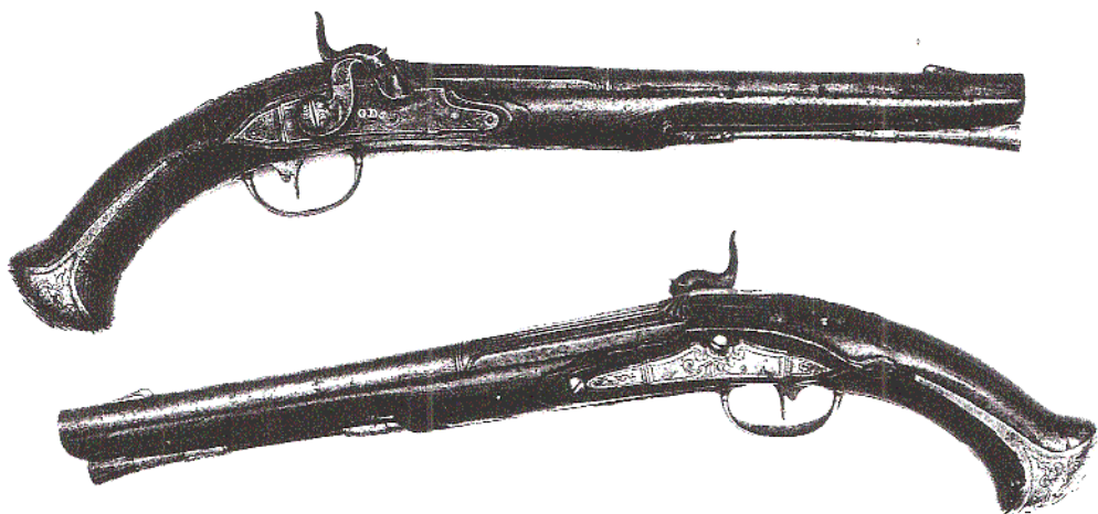
Ett par slagläspistoler, ändrade från flintläs, signerade GDS. Total längd 45 cm. Pipornas längd 28 cm, slätborrade. Beslag av järn. Kaliber 14 mm. (Privat ägo)
