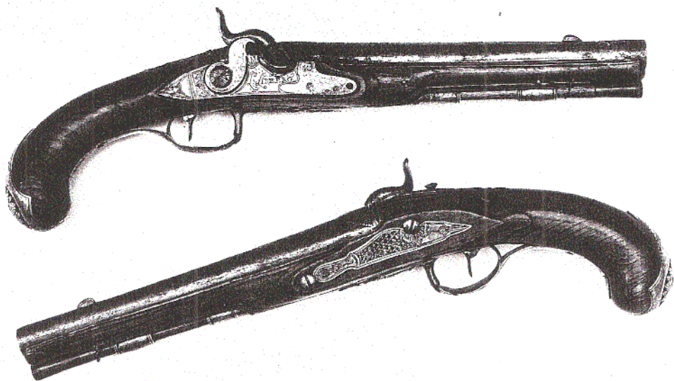
Ett par slaglåspistoler, ändrade från flintlås, signerade L:LIDBERG. Total längd 36,5 cm. Pipornas längd 21,5 cm, slätborrade. Beslag av mässing. Kaliber 14 mm. (Privat ägo)
