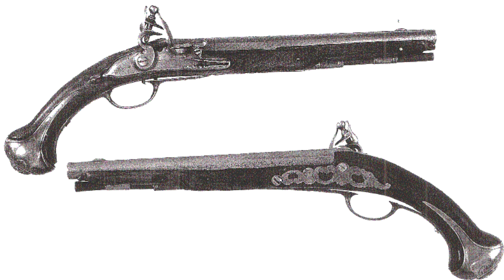
Ett par flintlåspistoler, signerade E:HOFVENSKIÖLT. Total längd 45 cm. Pipornas längd 27,5 cm, slätborrade. Beslag av mässing. Kaliber 15 mm. (Privat ägo)
