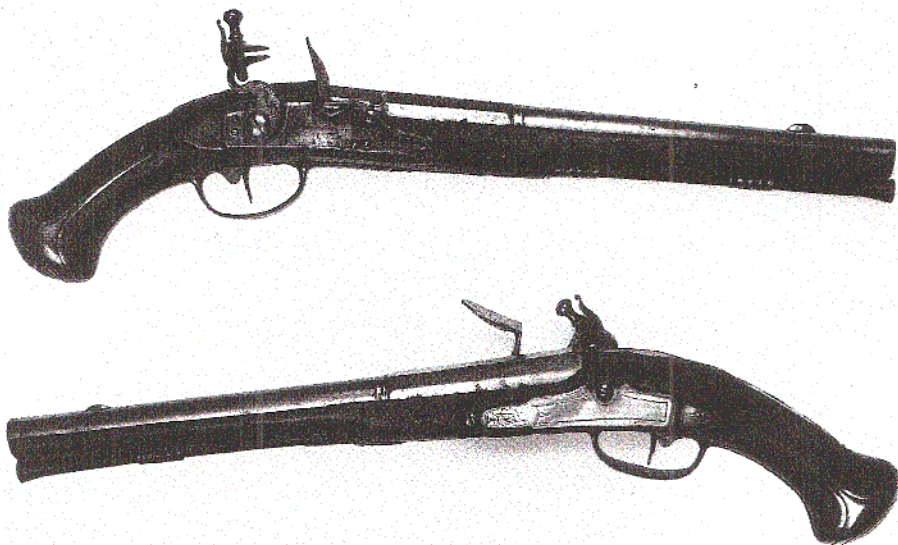
Ett par flintlåspistoler, signerade DAHLSTEDT ÖREBRO. Total längd 45,5 cm. Pipornas längd 30 cm, slätborrade. Beslag av mässing. Kaliber 15 mm. (Jönköpings läns museum)
