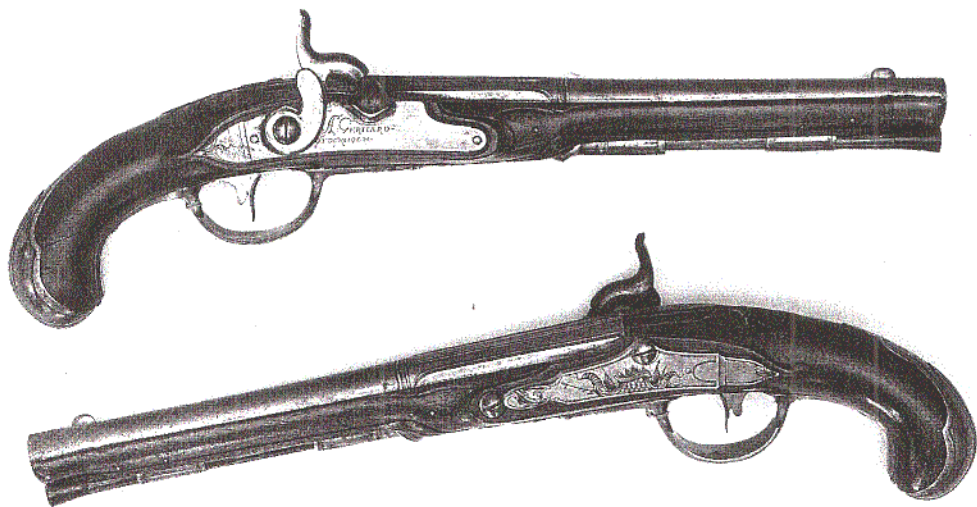
Ett par slagläspistoler, ändrade från flintläs, signerade A:GERHARD STOCKHOLM. Total längd 42 cm. Pipornas längd 27 cm, räfflade. Beslag av järn. Kaliber 14 mm. (Privat ägo)
