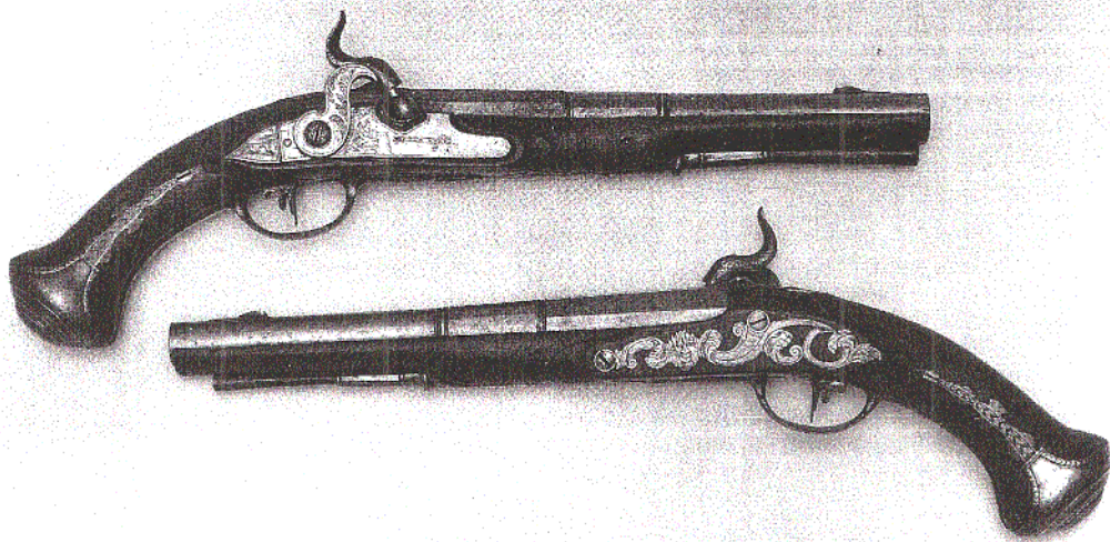
En par slaglåspistoler, ändrade från flintlås, signerade PETTER MÅRD. Total längd 44 cm. Pipornas längd 31 cm, slätborrade. Beslag av järn. Kaliber 15 mm. (Privat ägo)
