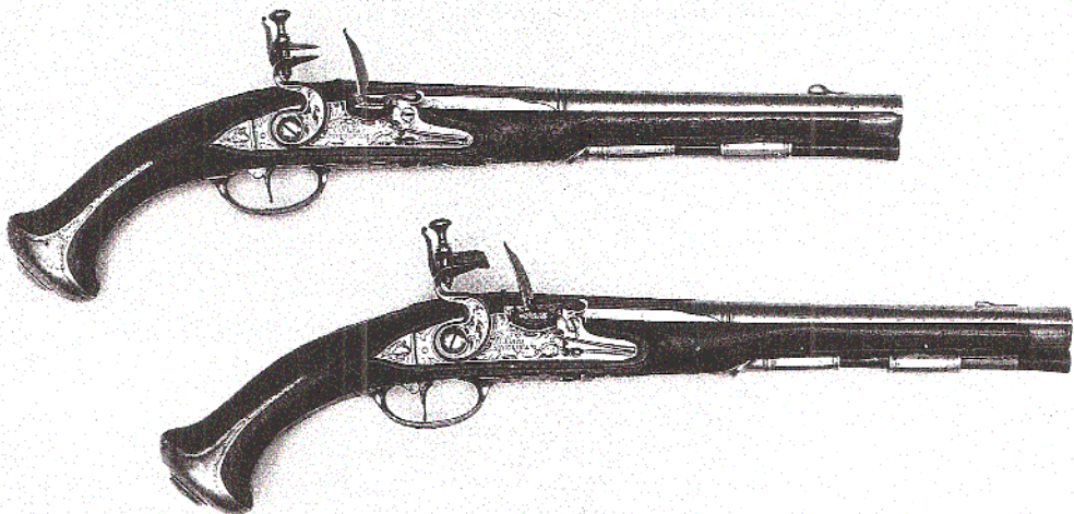
Ett par flintlåspistoler, signerade D:BARS STOCKHOLM. Total längd 44 cm. Pipornas längd 28 cm, slätborrade. De är signerade D:BARS i guld. Beslag av järn. Kaliber 14 mm. (Privat ägo)
