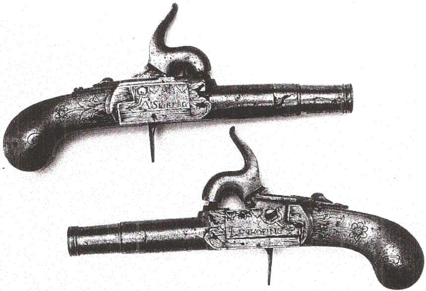
Ett par slaglåspistoler, ändrade från flintlås, signerade A:SIÖBERG LINKÖPING. Total längd 15 cm. Vapnen är tillverkade helt i stål. Kaliber 12 mm. (Privat ägo)
