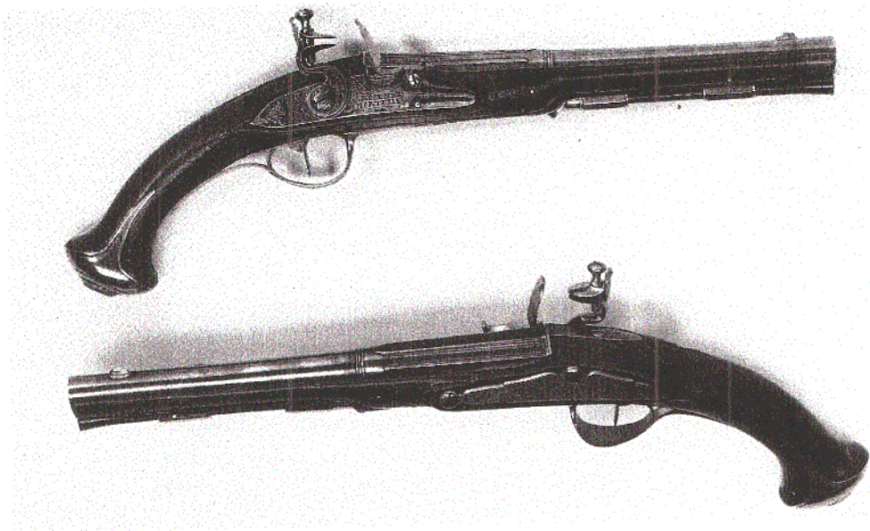
Ett par flintlåspistoler, signerade J:ROSENEL NORTELIE. Total längd 38 cm. Pipornas längd 23 cm, slätborrade. Beslag i järn. Kaliber 13 mm. (Privat ägo)
