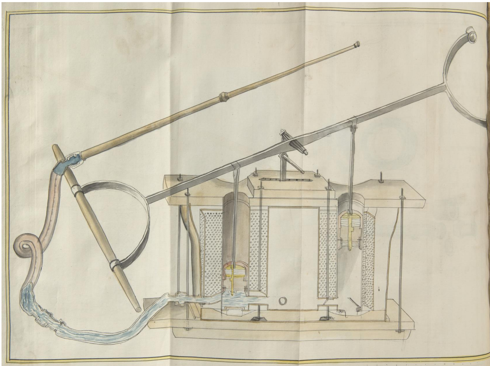
Профиль пожарного насоса 25
